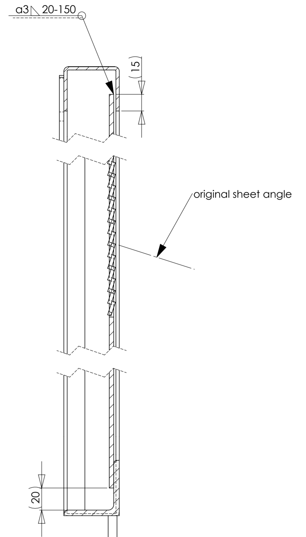
SECTION D-D SCALE 1 : 2
