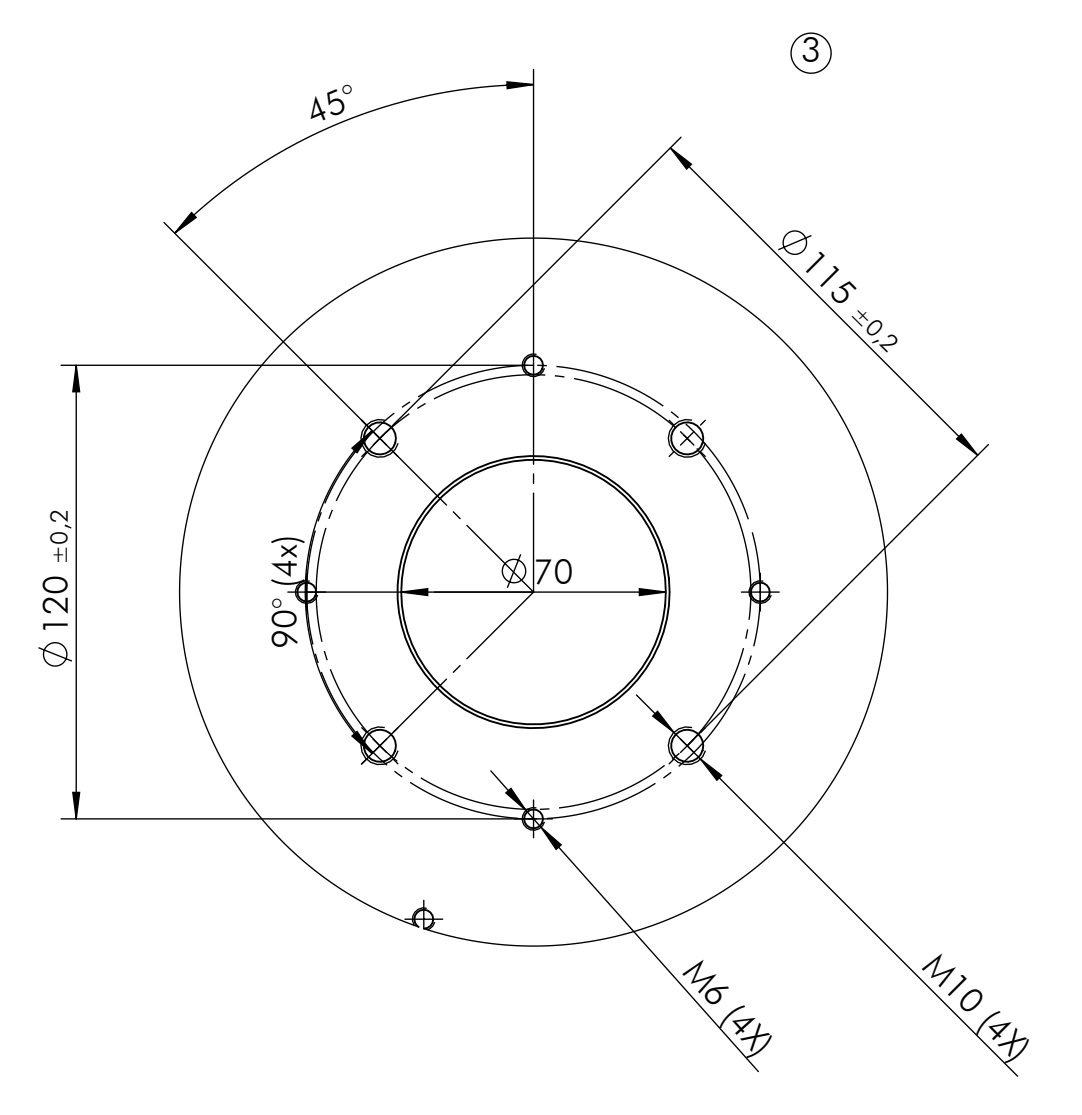
F (1 : 2) (2X)
