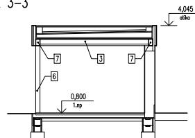
ŘEZ 3-3
