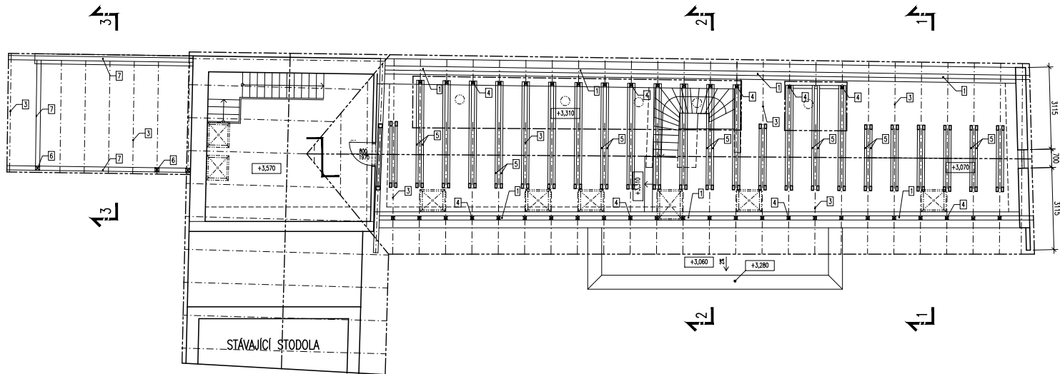
ŘEZ 1-1
