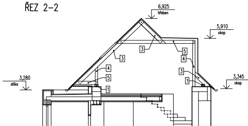
ŘEZ 2-2
