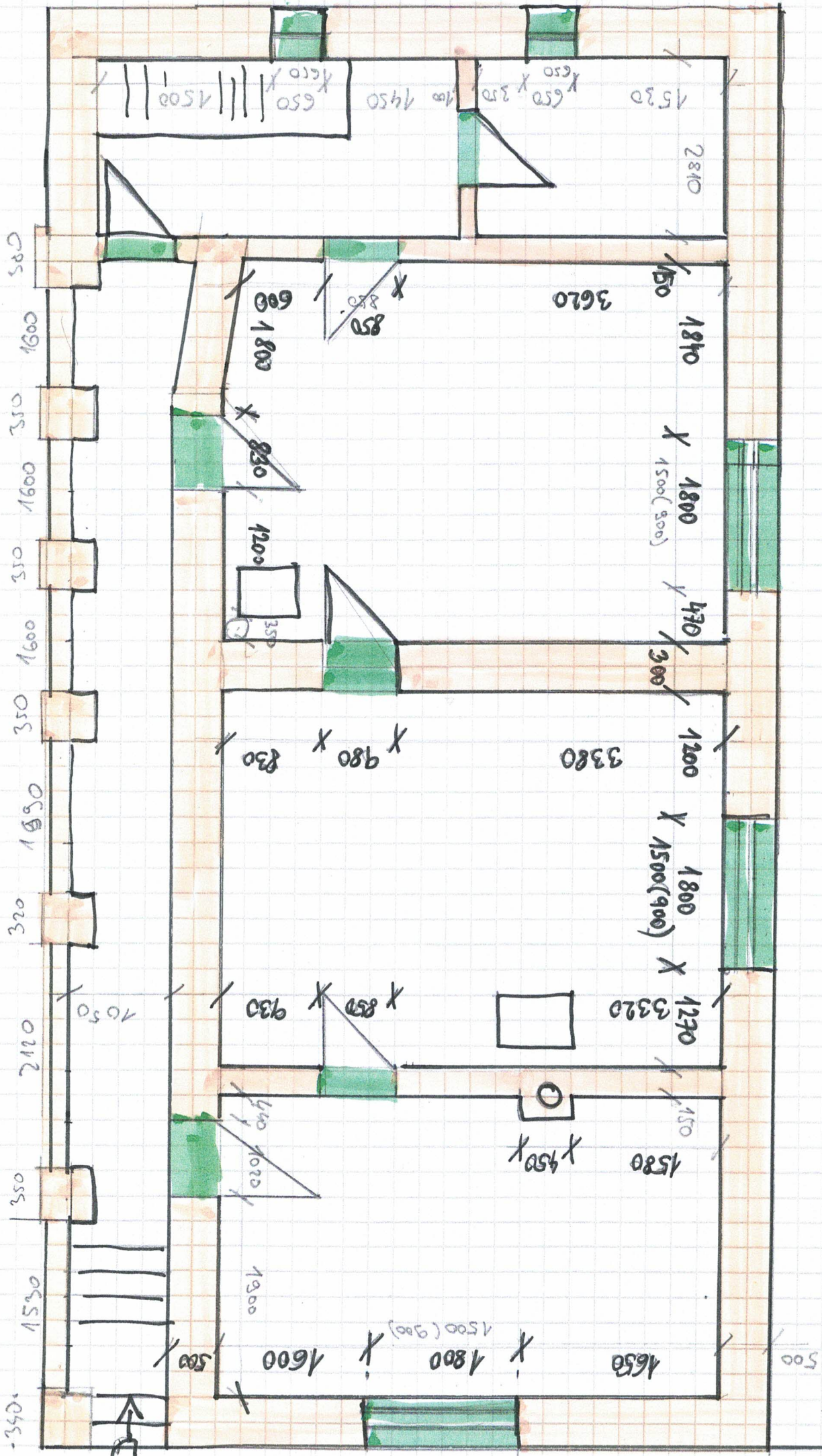
FIGAS 16 (1. poschodie)
