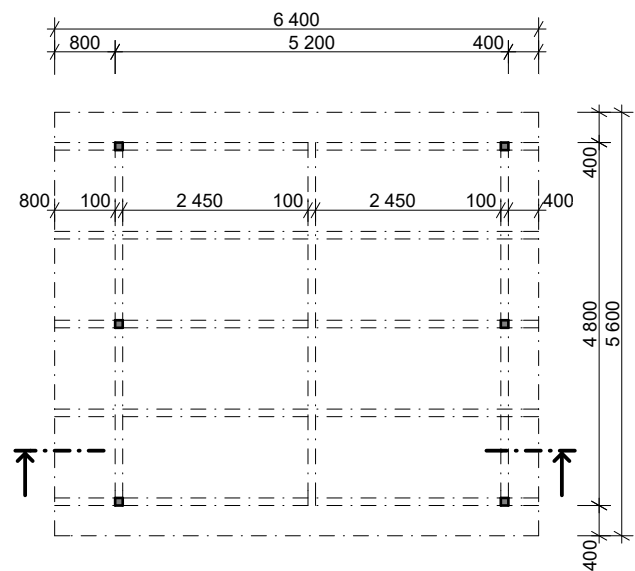
PÔDORYS, M 1:100
