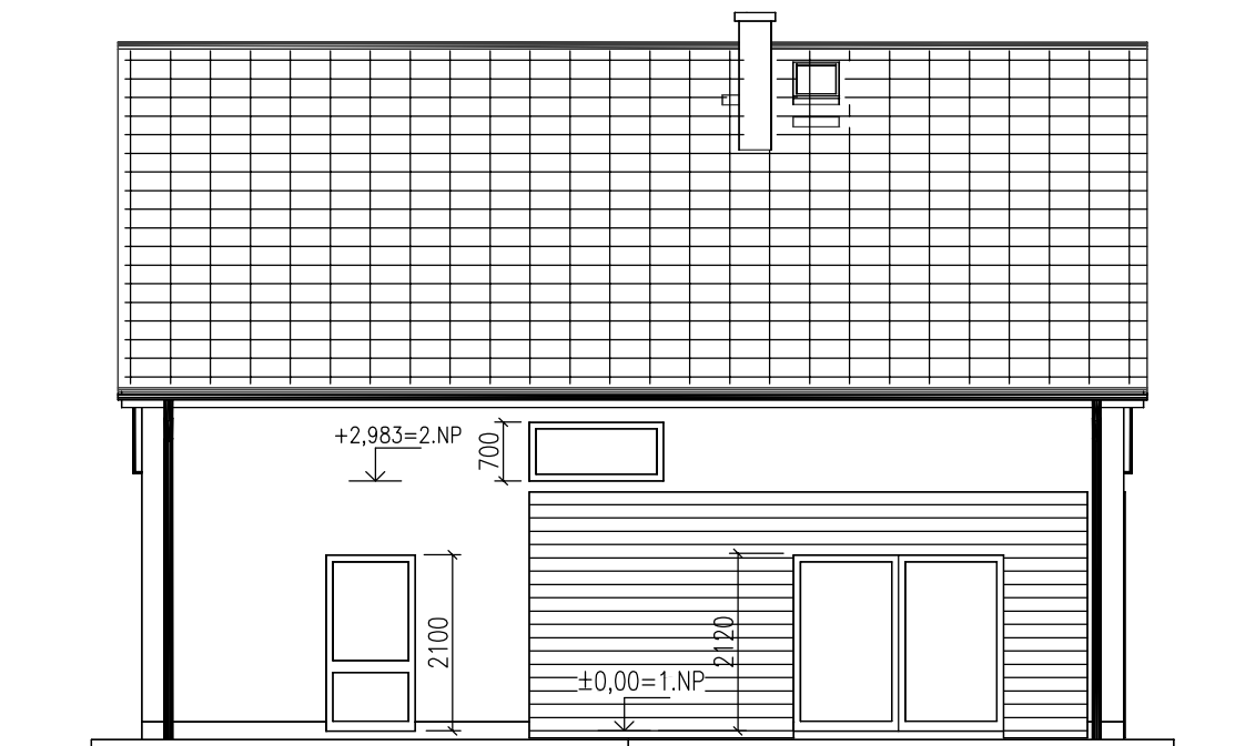
POHLED JIHOZÁPADNÍ
