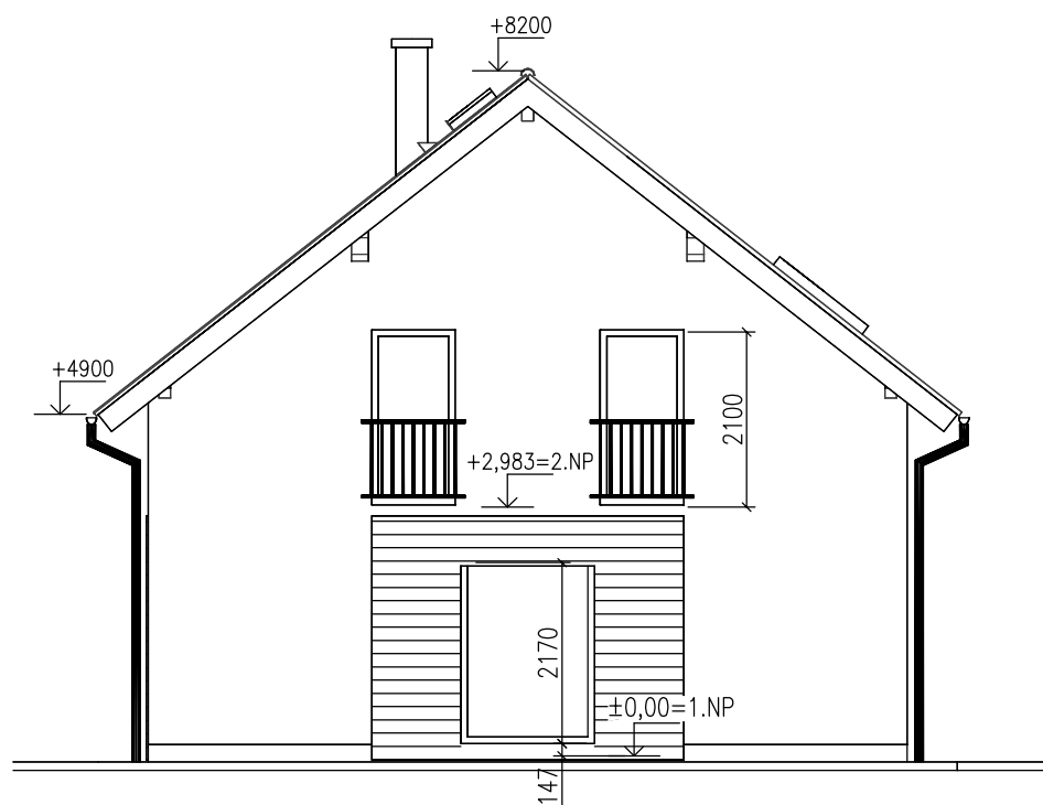
POHLED JIHOVÝCHODNÍ
