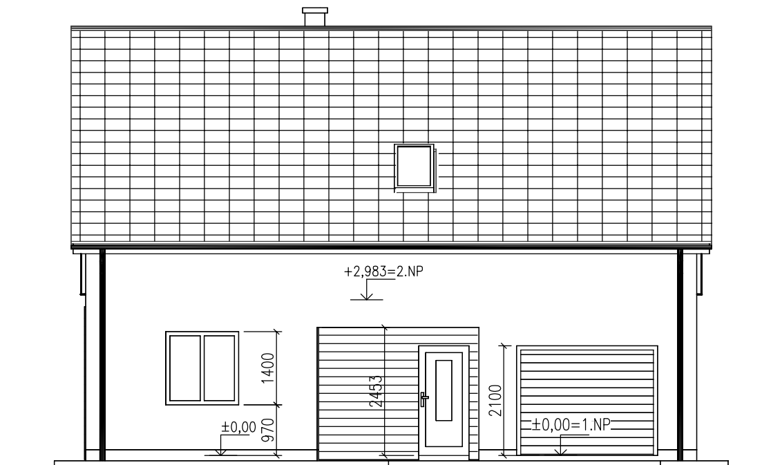
POHLED SEVEROVÝCHODNÍ
