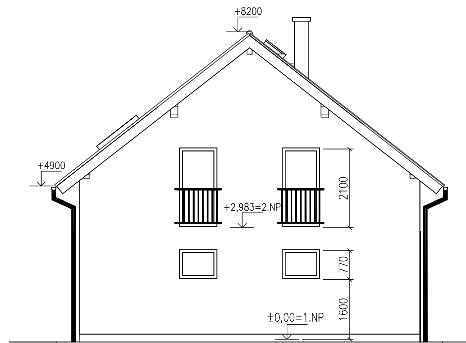
POHLED SEVEROZÁPADNÍ
