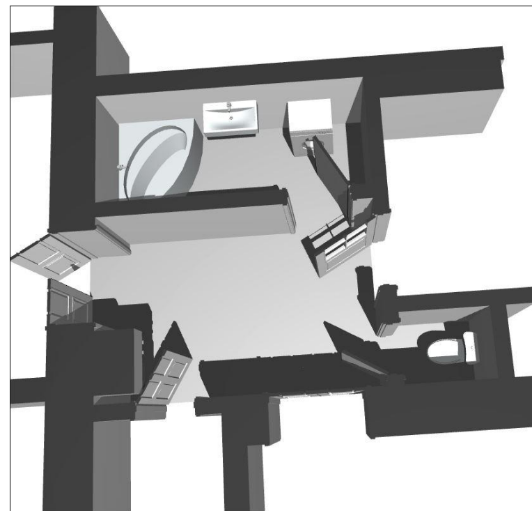
PERSPEKTIVNÍ SCHEMA
