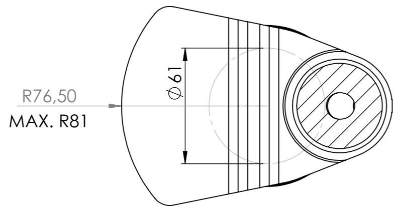
ŘEZ C-C MĚŘITKO 1 : 2
