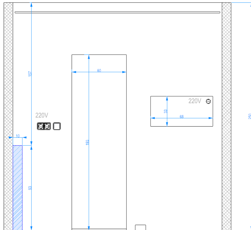
Pohled D
