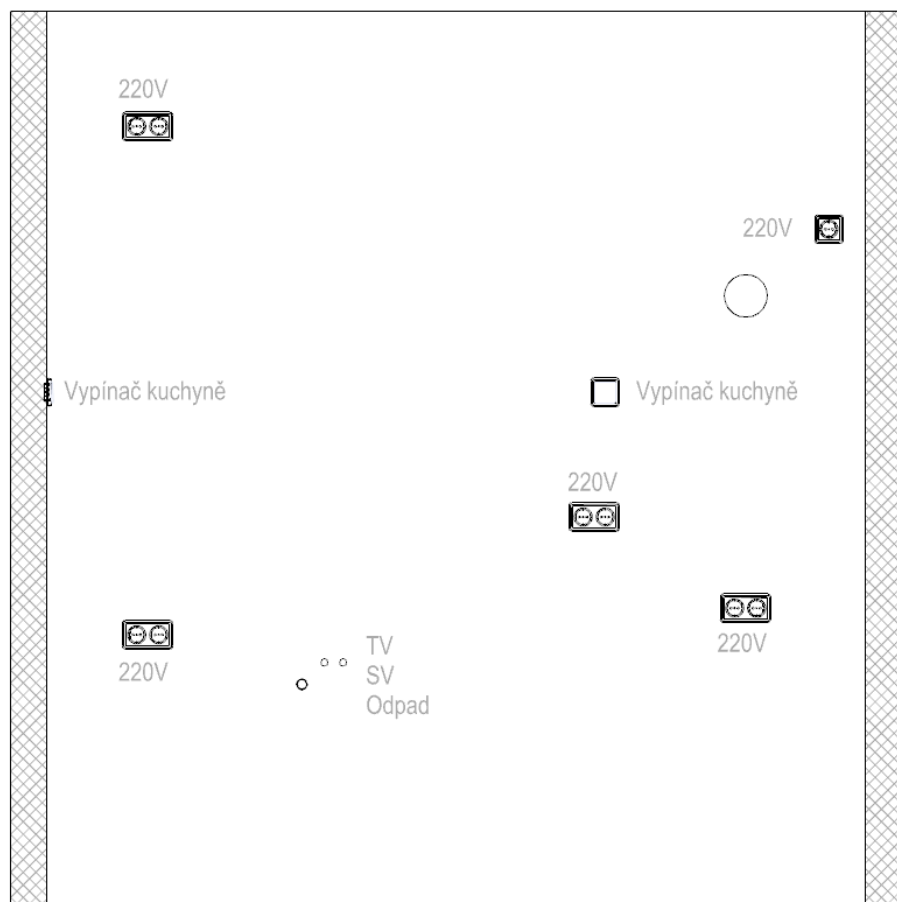
Pohled kuchyně
