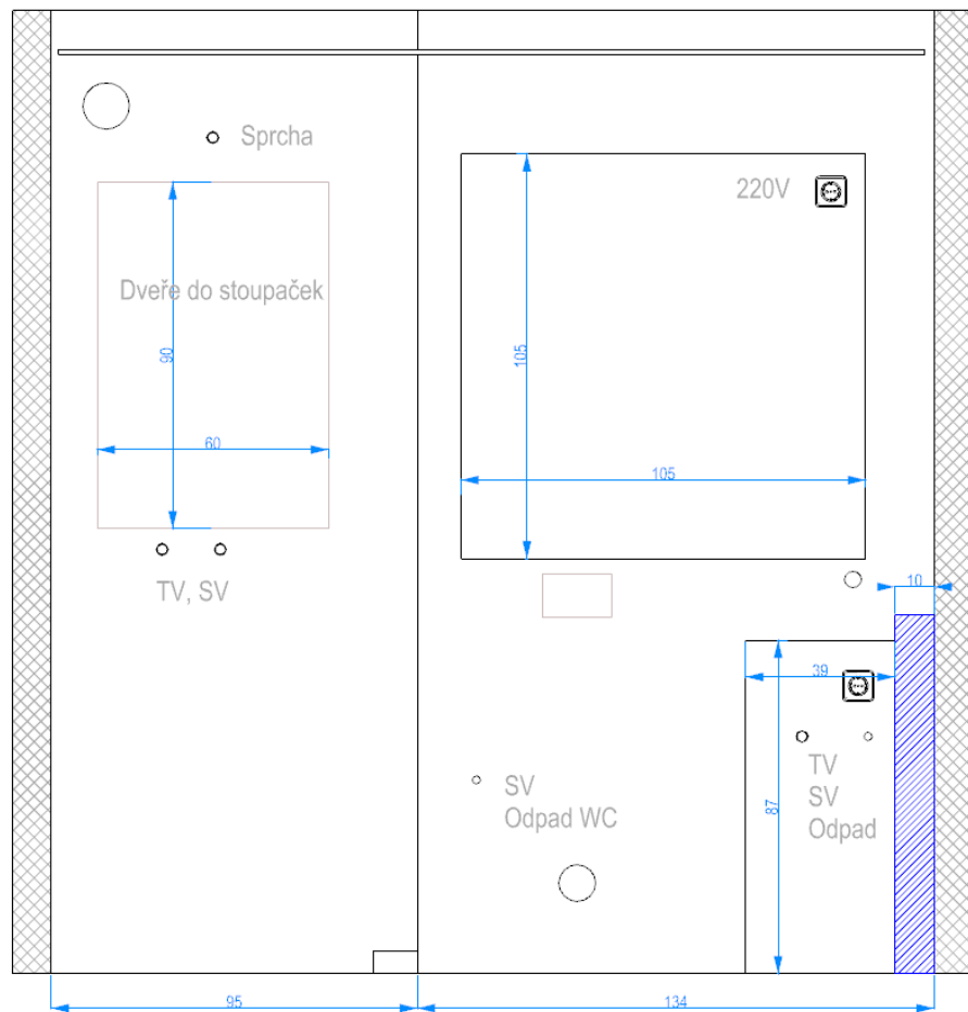
Pohled A
