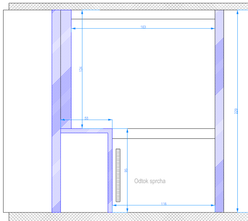
Půdorys
