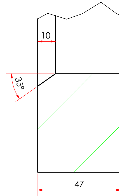
B (1 : 1)
