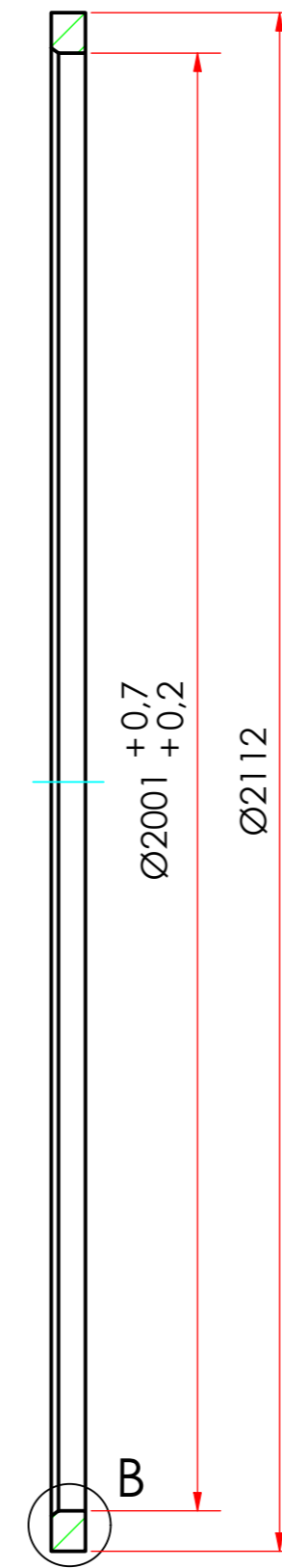
A-A (1 : 10)
