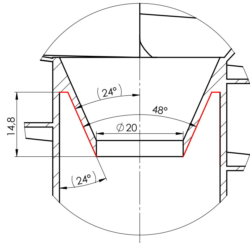
DETAIL E MĚŘITKO 2 : 1
