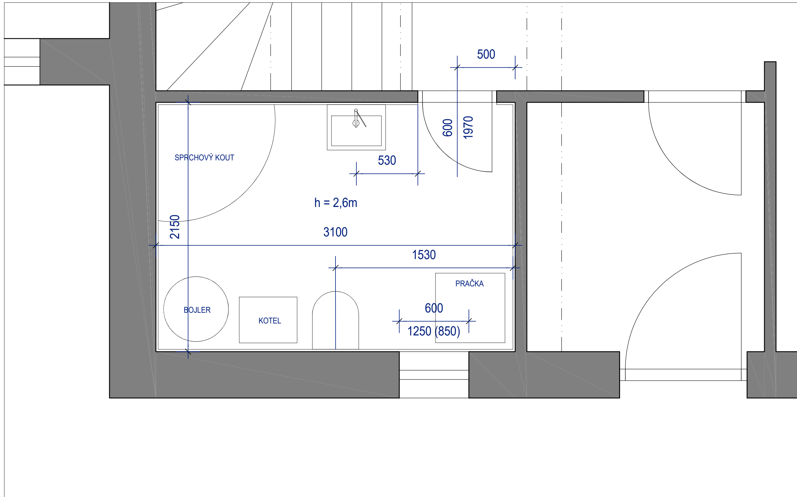
SPODNÍ KOUPELNA M 1:20
