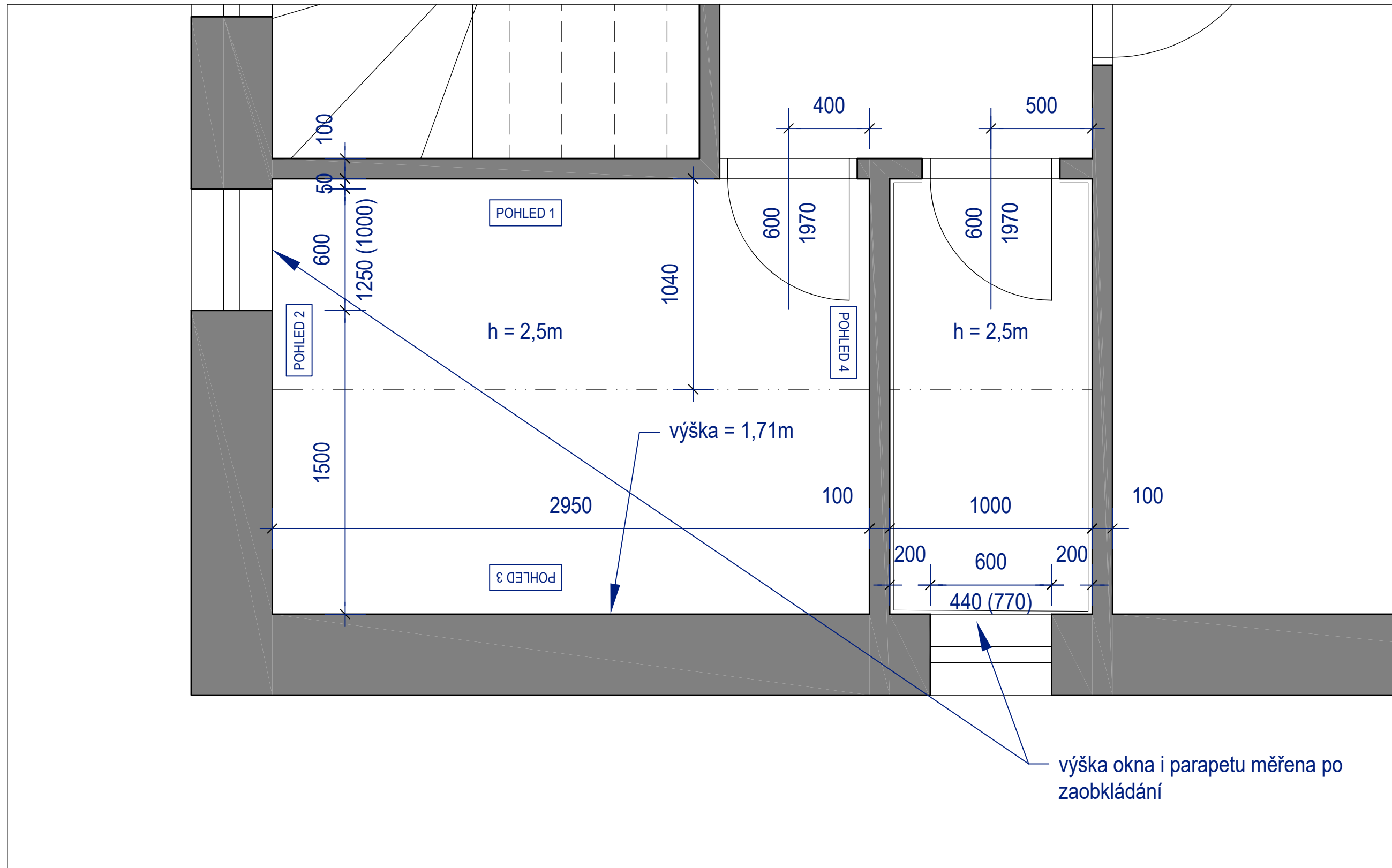
HORNÍ KOUPELNA A WC M 1:20
