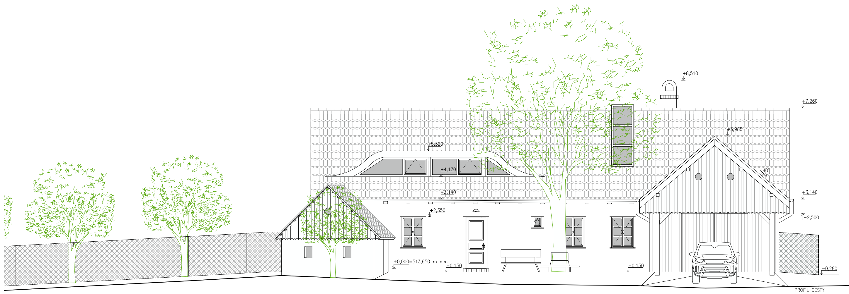
ZÁPADNÍ POHLED
