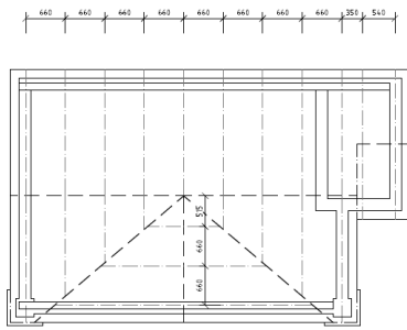
PŮDORYS KROVU
