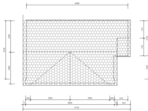
PŮDORYS STRECHY
