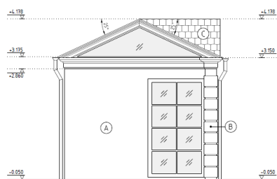
POHLED JUŽNÝ
