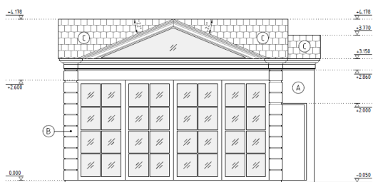
POHLED VÝCHODNÝ
