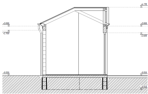
PRIEČNY REZ
