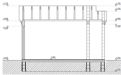
POZDĽŤNY REZ
