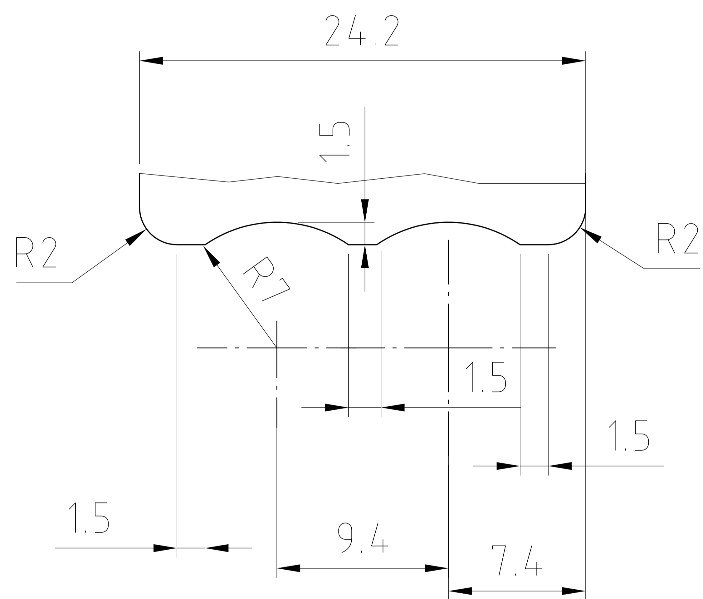
Ansicht X
