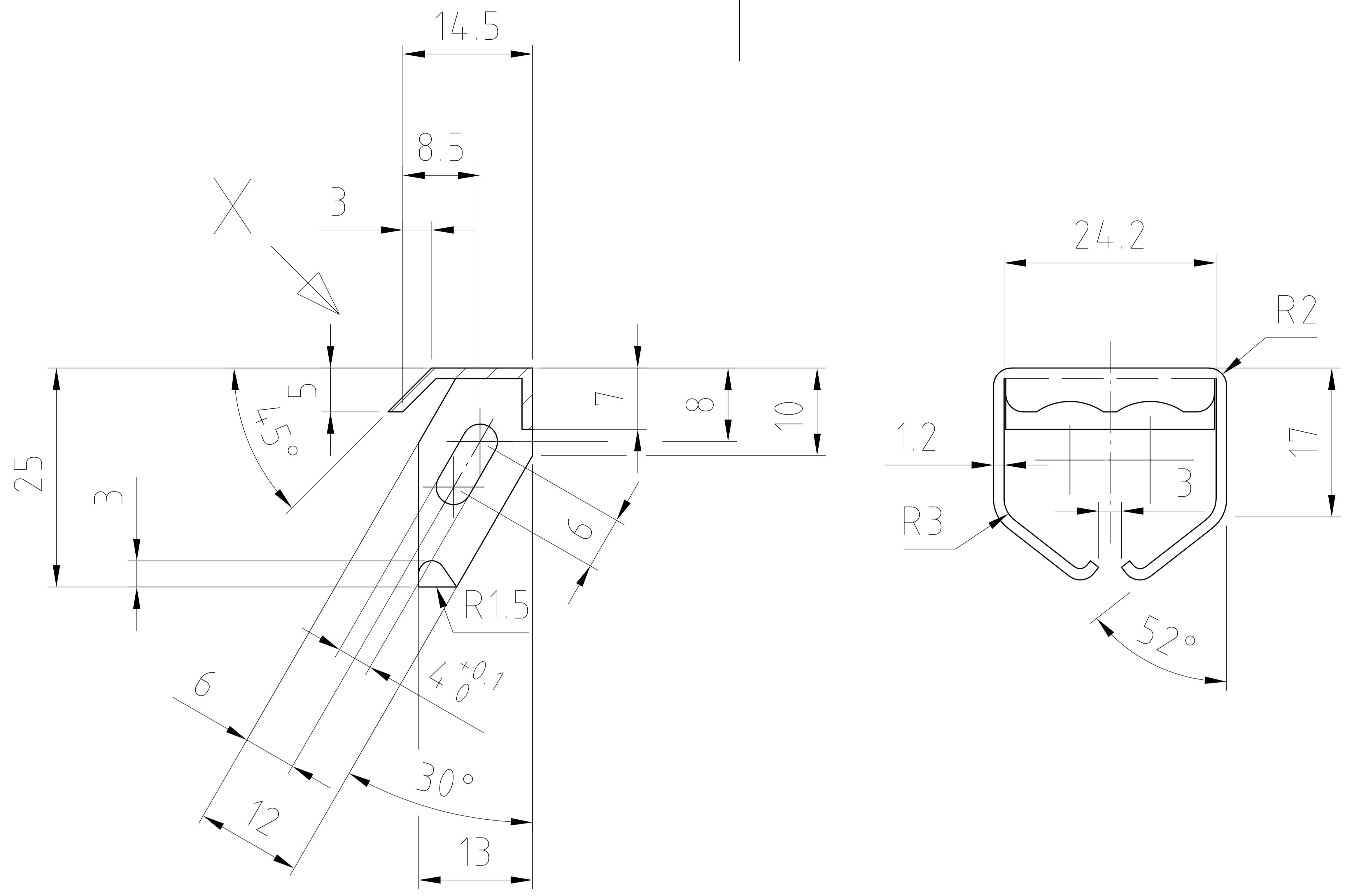
Ansicht X
