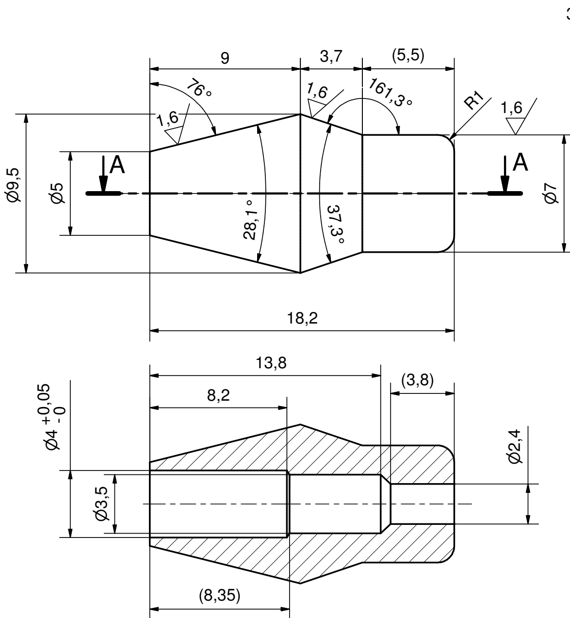
A-A (5:1)
