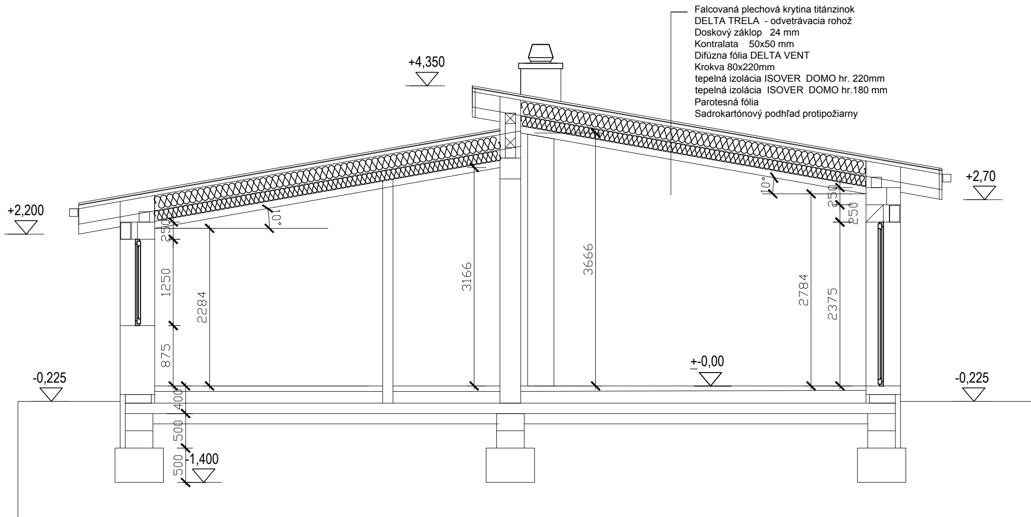
REZ A - A 1 : 100
