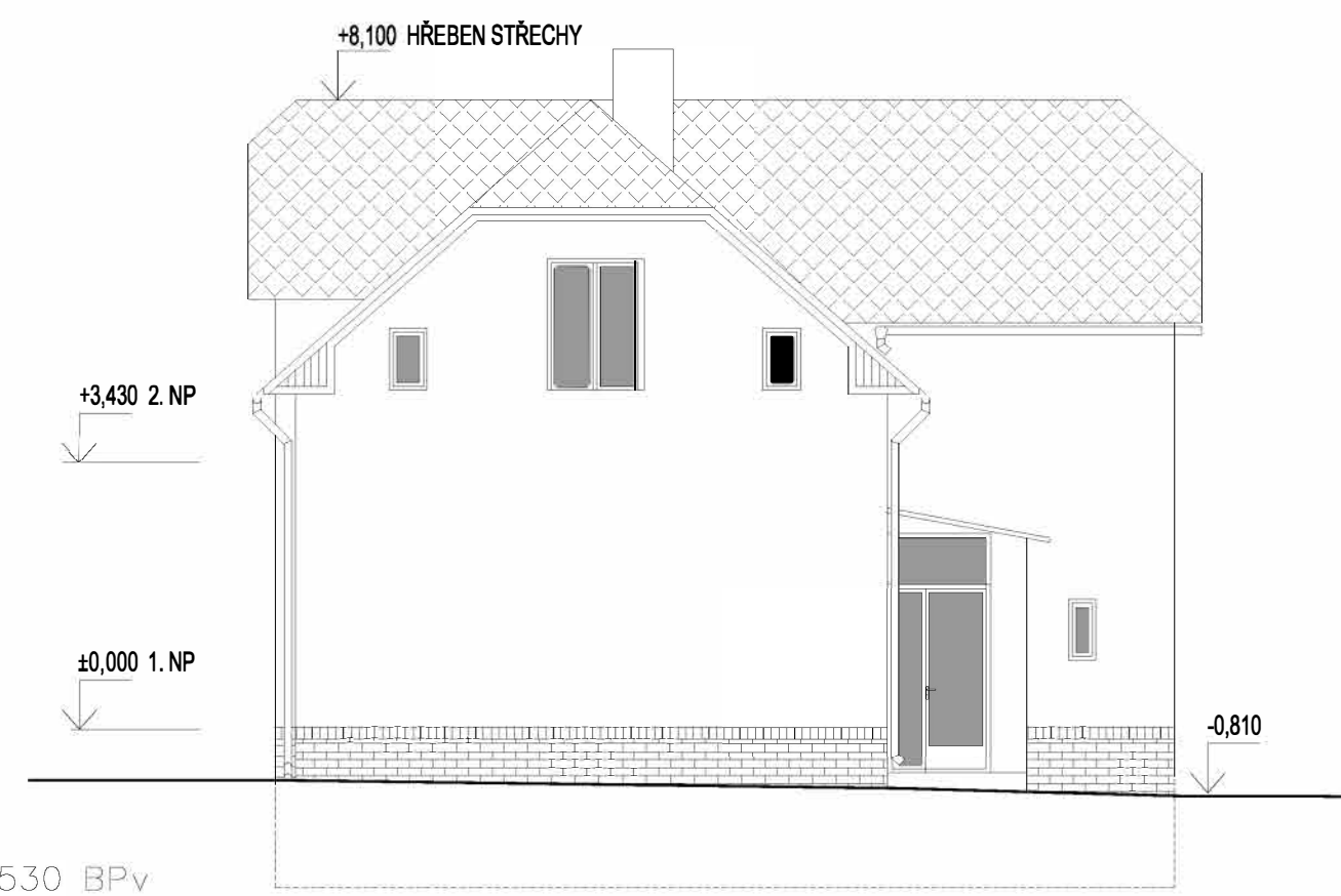
POHLED JIHOVÝCHODNÍ
