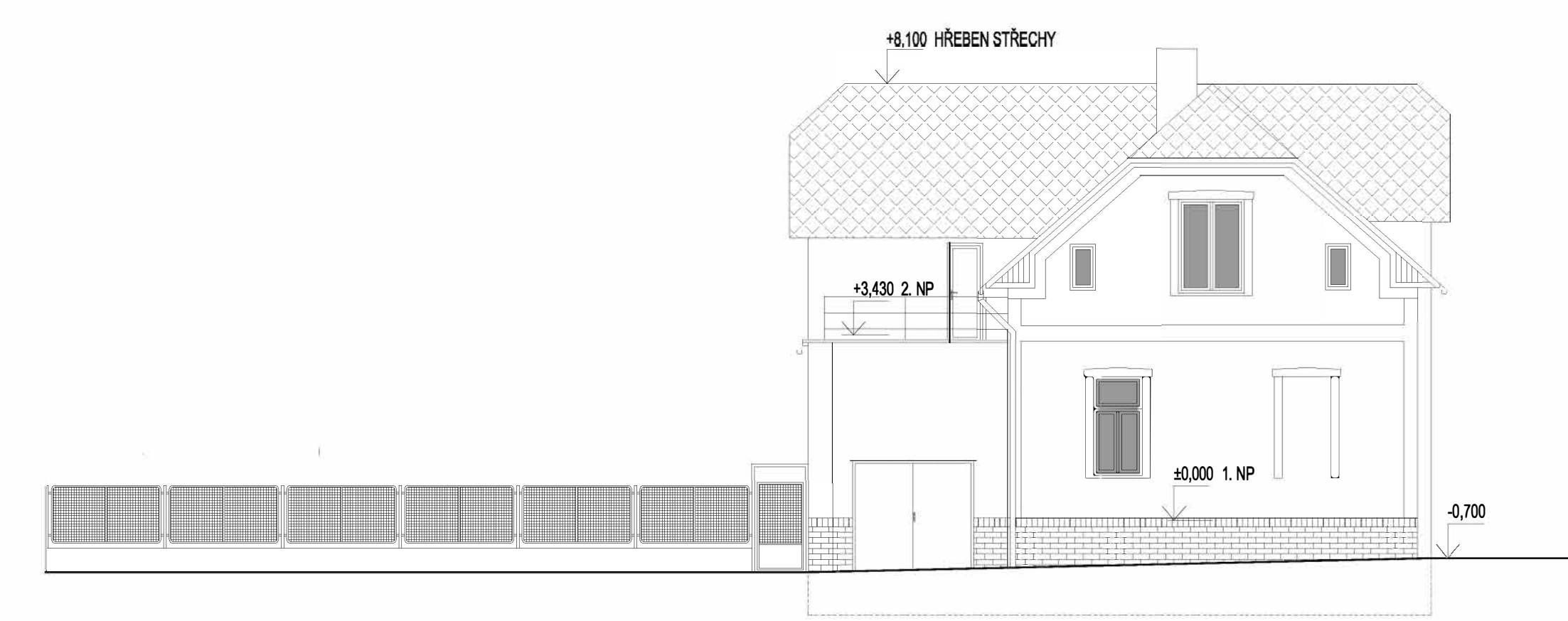
POHLED SEVEROZÁPADNÍ
