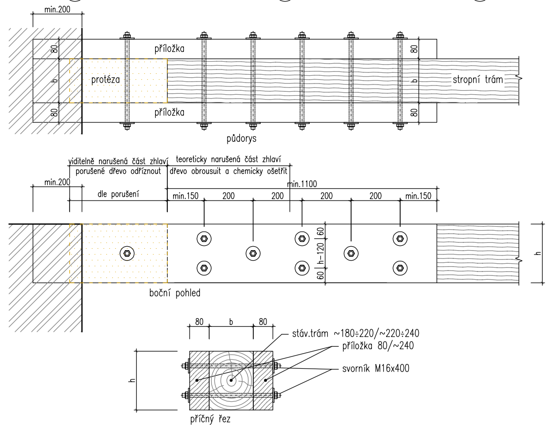
DETAIL PŘÍLOŽEK STROPNÍHO TRÁMU M 1:15
