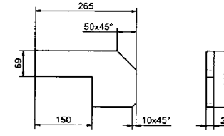
0005285-S07 (1:5)
