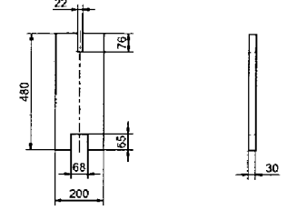
0005285-S05 (1:10)
