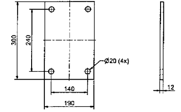
0005285-S04 (1:5)
