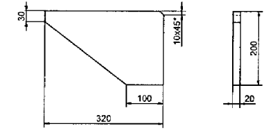
0005285-S06 (1:5)
