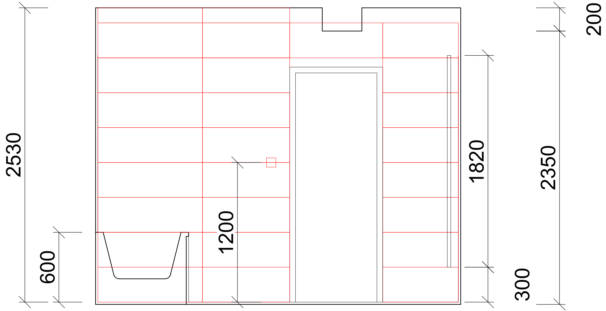
POHLED NA STĚNU S DVEŘMI
