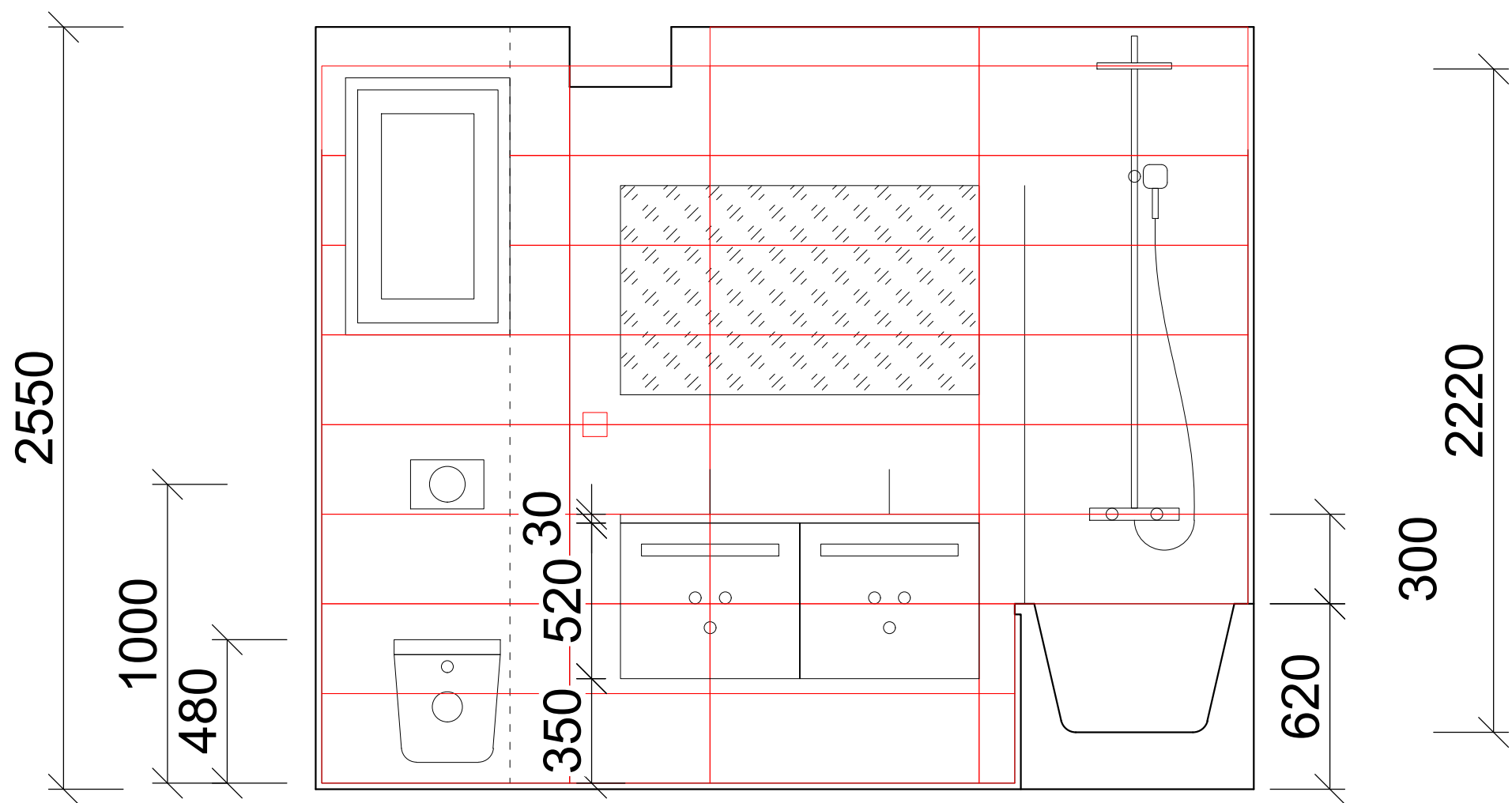
POHLED NA STĚNU S UMYVADLEM
