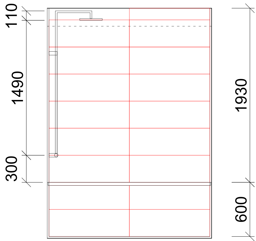
POHLED NA STĚNU S VANOU
