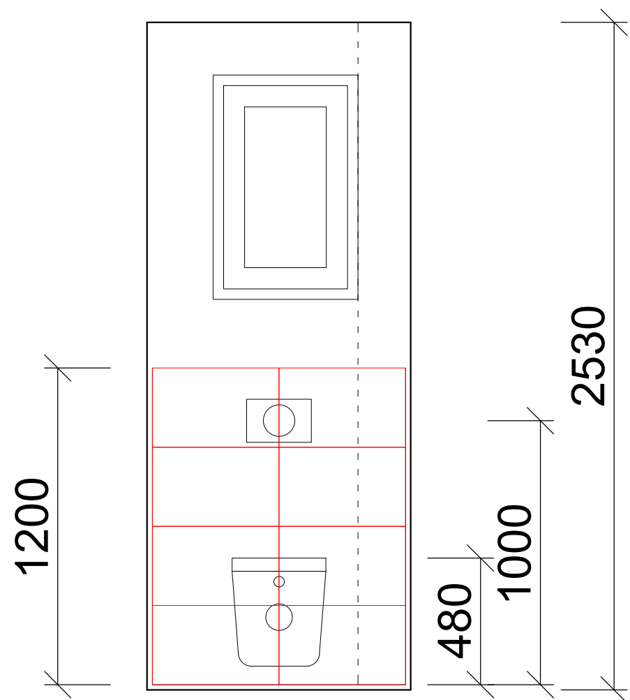
POHLED NA STĚNU S WC
