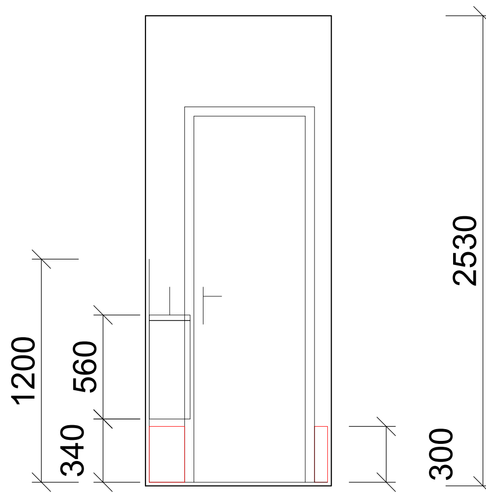
POHLED NA STĚNU S DVEŘMI
