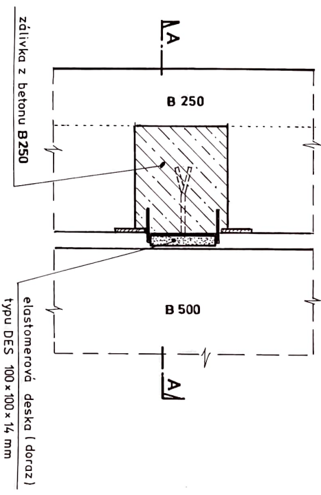
- půdorysný řez B-B M 1:5
