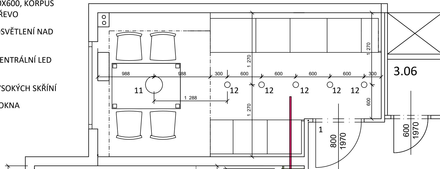
KUCHYNĚ - SCHÉMA SVÍTIDEL
