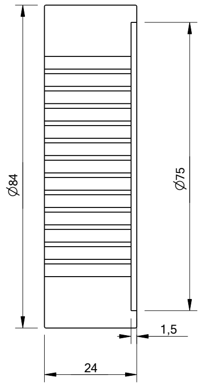
Section A-A
