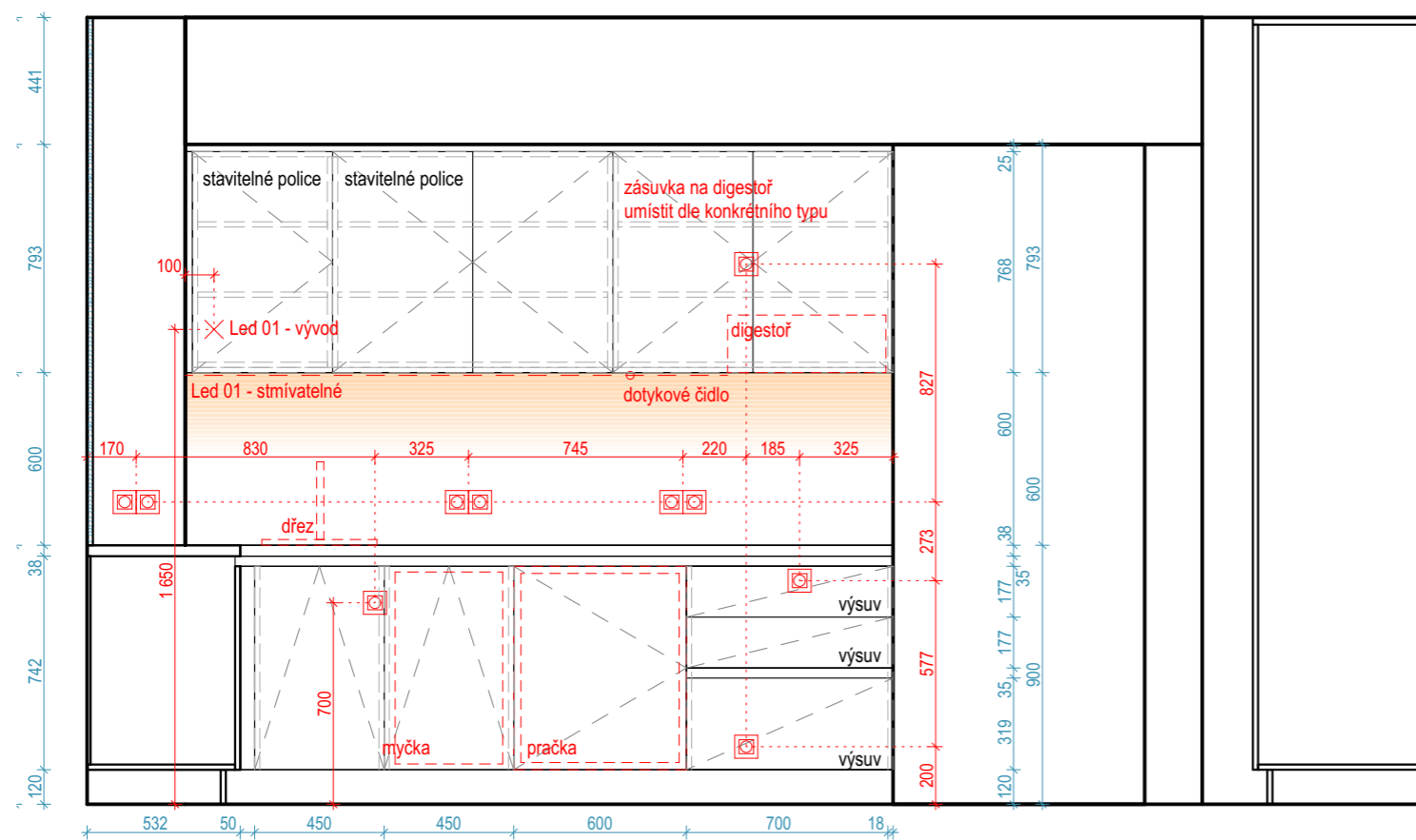
AN.01 - Pohled 2 - M1:25
