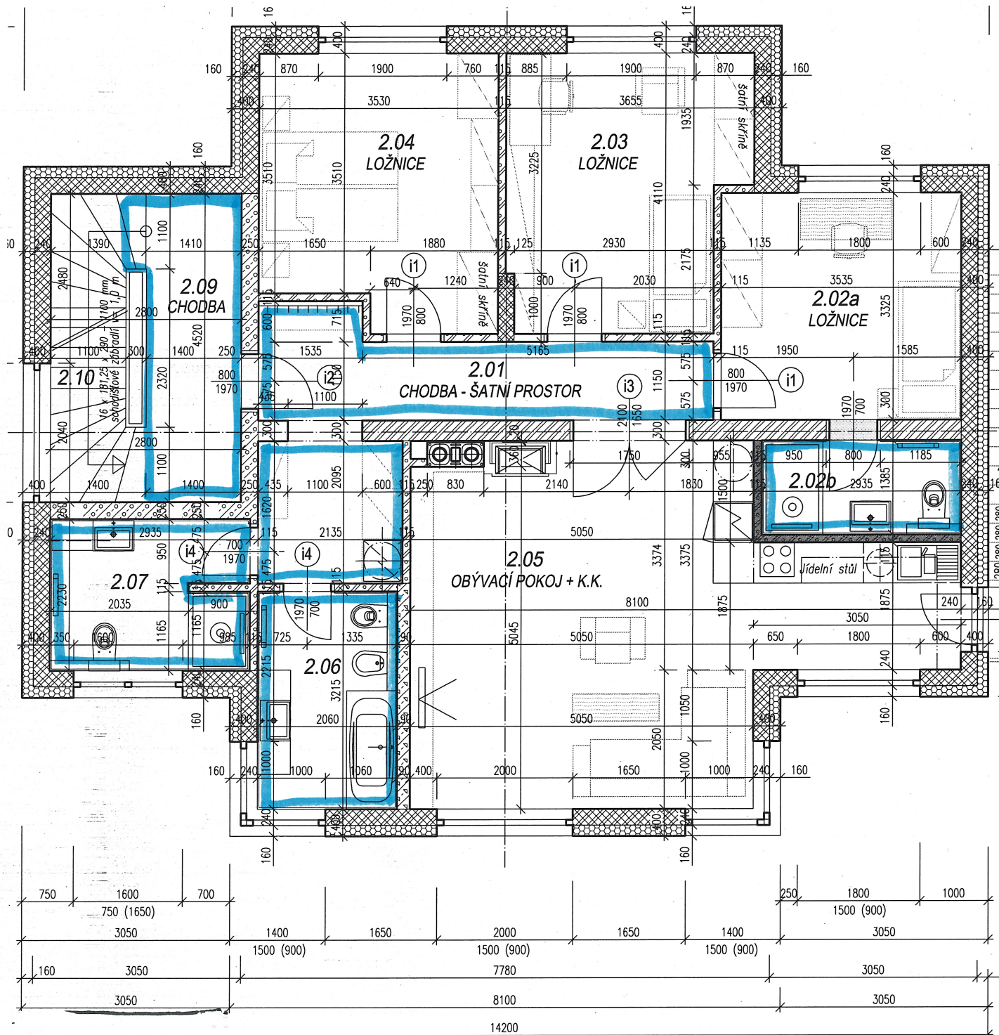
1. TABULKA MÍSTNOSTÍ 2. NP - pohledy SDK, 2.07, 2.06, 2.02b - vodorovný sdk
