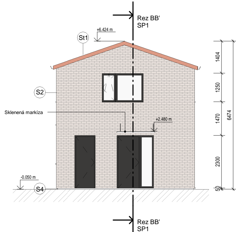
Pohľad - D1
