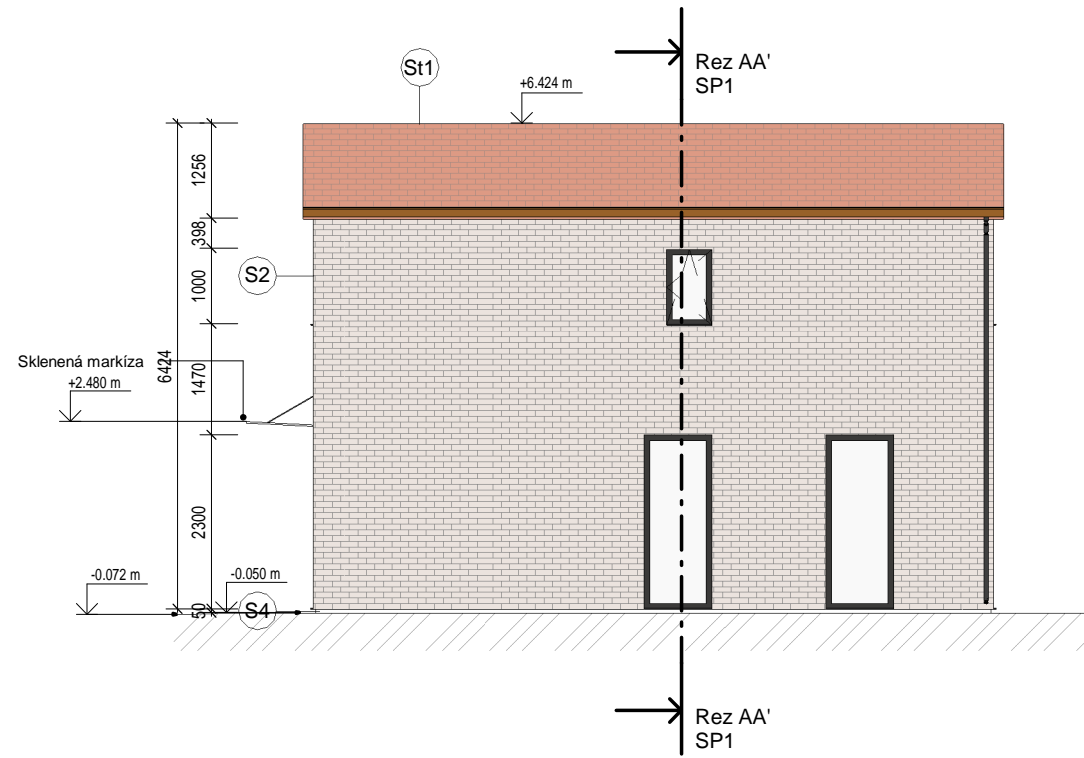
Pohľad - A1
