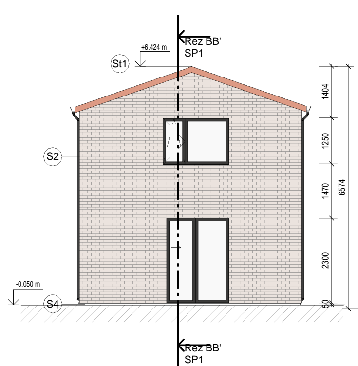
Pohľad - C1
