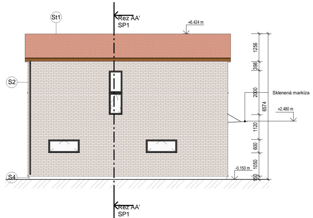
Pohľad - B1
