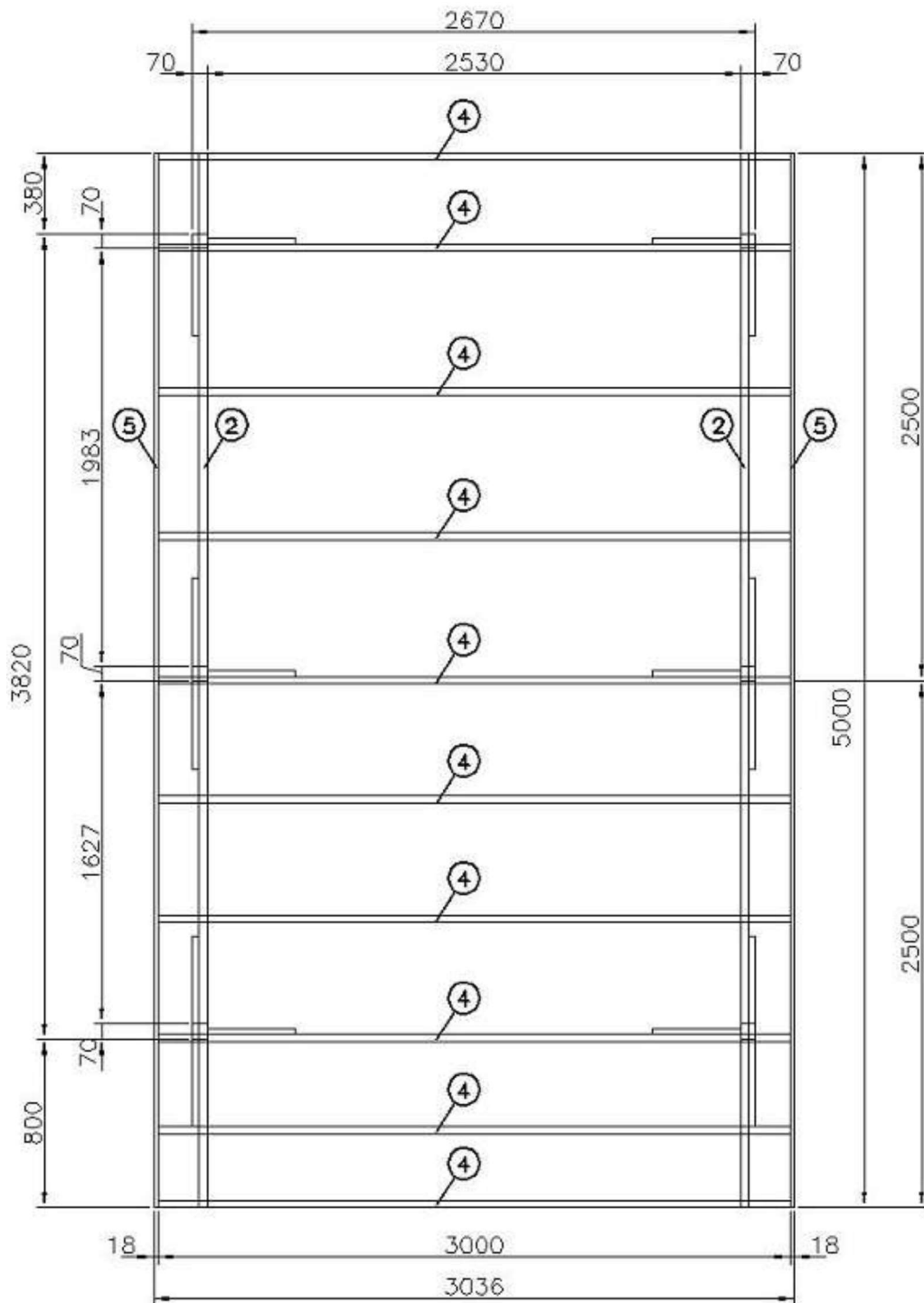
SÚPIS DIELOV PRE CARPORT ECONO V20.0
