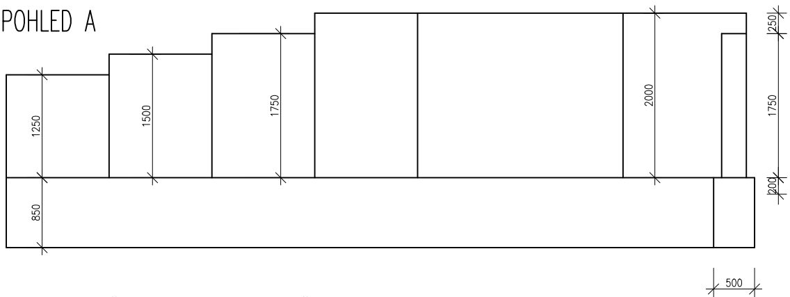
OPĚRKA ZE ZTRACENÉHO BEDNĚNÍ A ZÁKLADOVÉ DESKY, VŠE ARMOVÁNO
