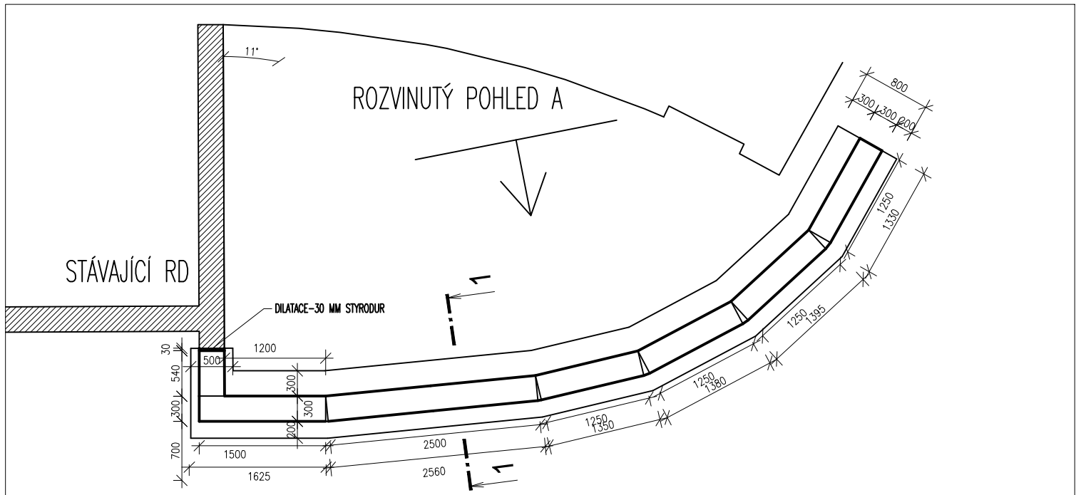
PŮDORYS
