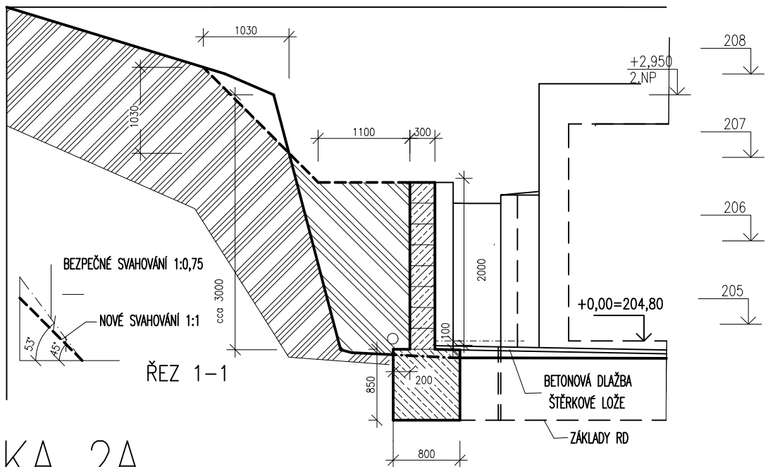
OPĚRKA ZE ZTRACENÉHO BEDNĚNÍ A ZÁKLADOVÉ DESKY, VŠE ARMOVÁNO
