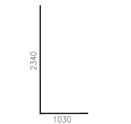
01 ∅16mm \bar{\alpha} 200mm CELKOVÁ DÉLKA 1ks 3370mm POČET 14ks
