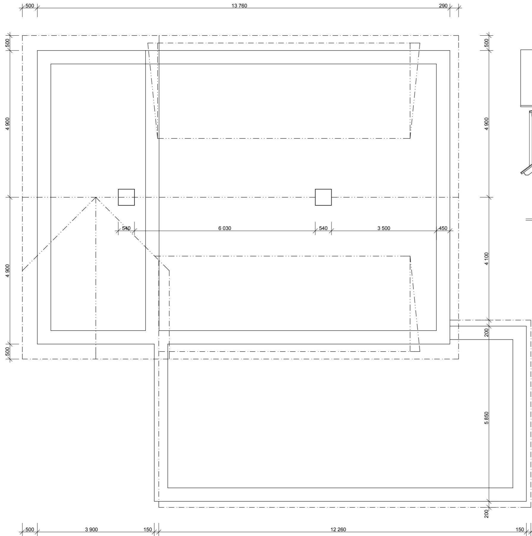
PŮDORYS STŘECHY :
