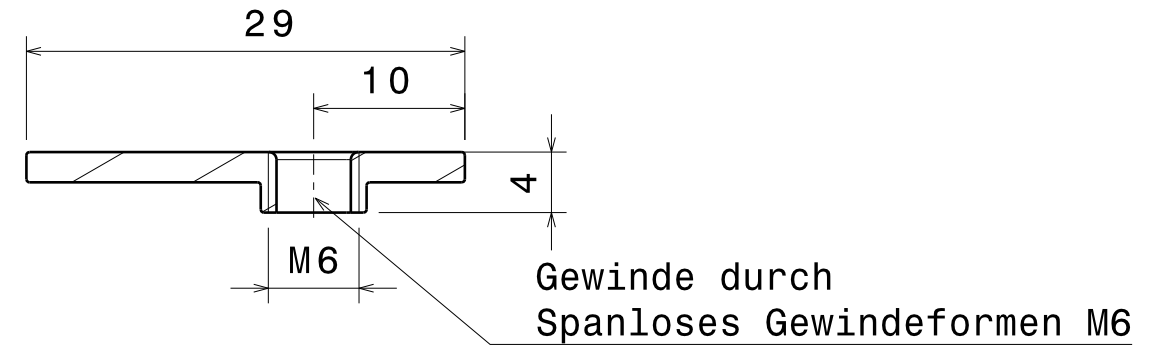
Schnitt A-A Maßstab: 2:1
