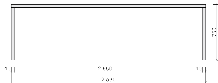
POHLED STŮL
