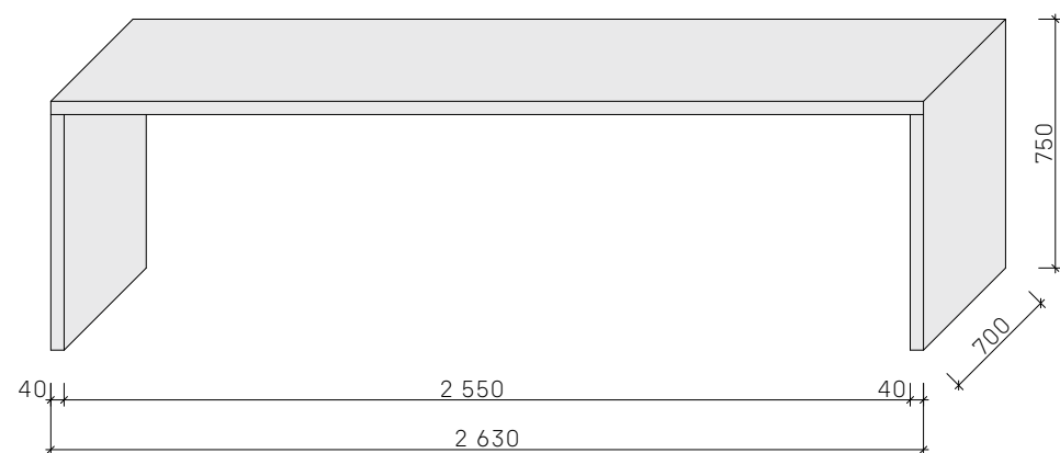
AXONOMETRIE STŮL
