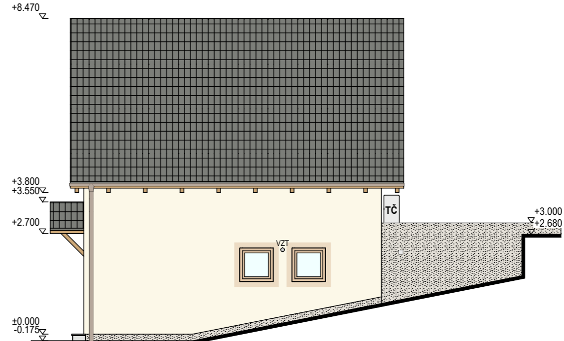
POHLED VÝCHODNÍ
