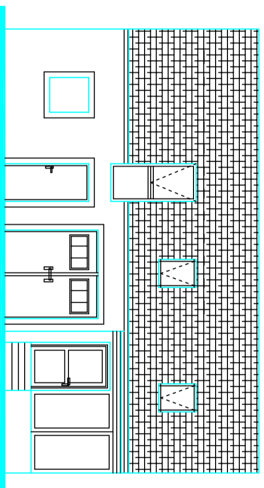
POHLED JIHOZÁPADNÍ
