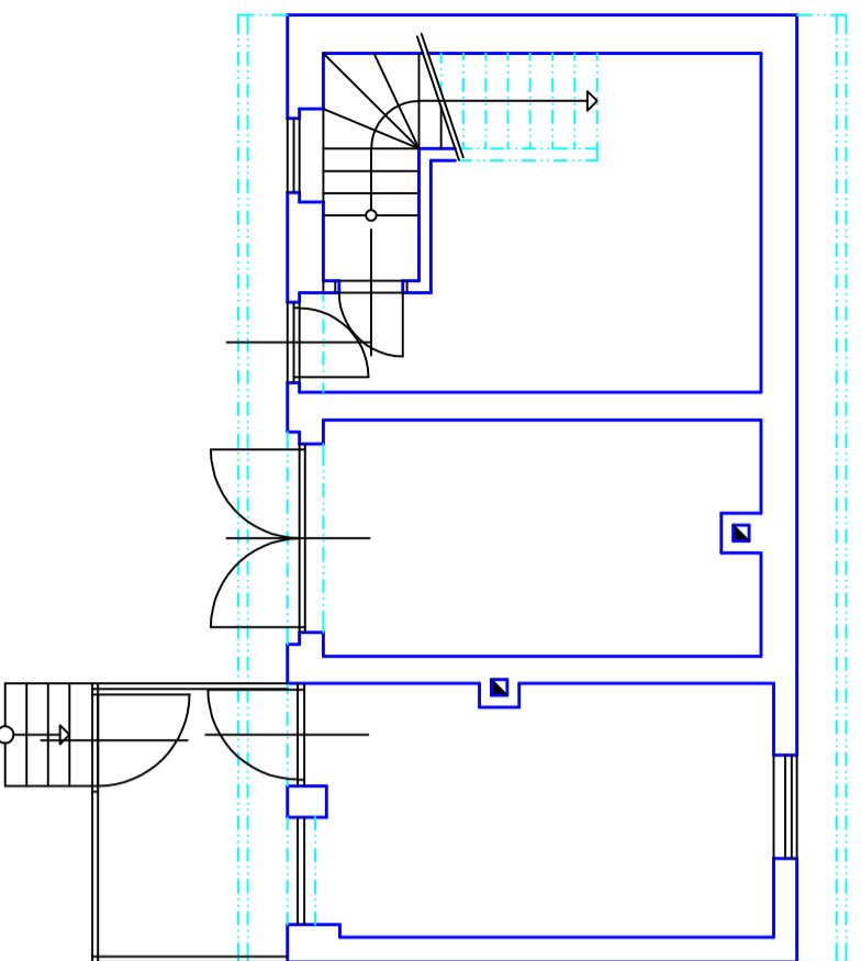
PŮDORYS I.NP
