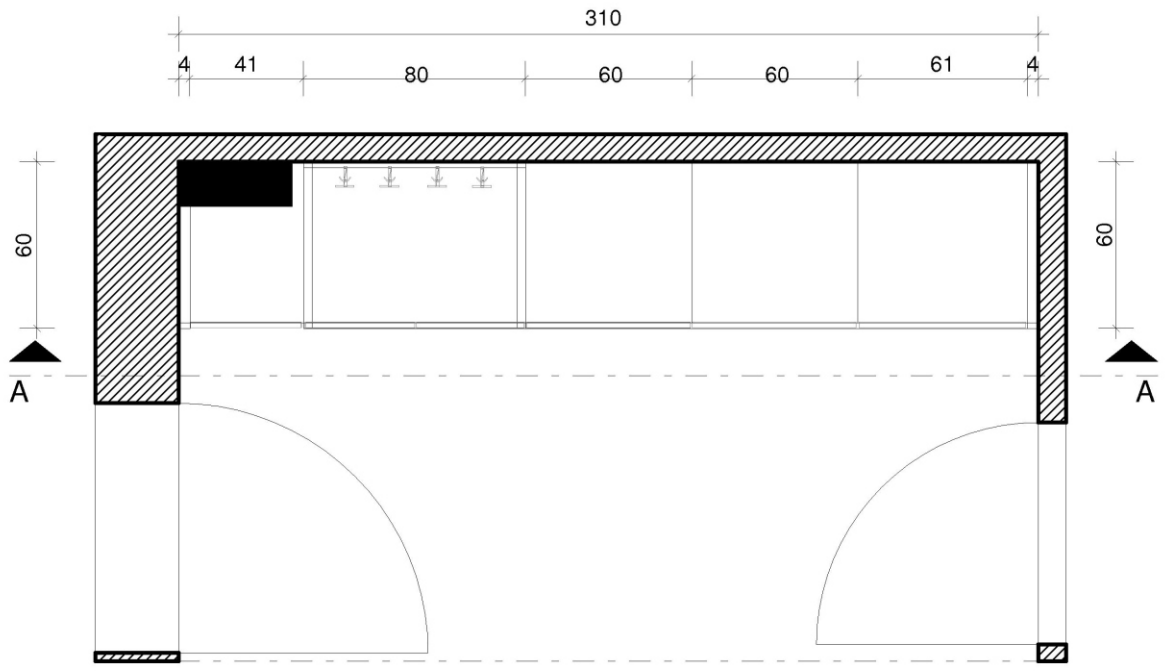
Řez A-A
