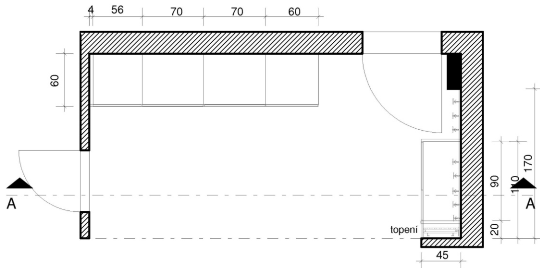
Řez A--A
