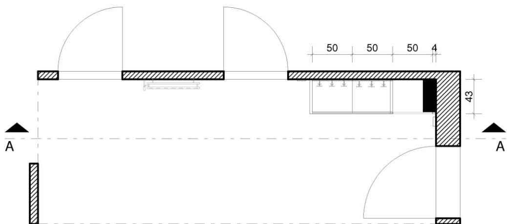
Řez A--A
