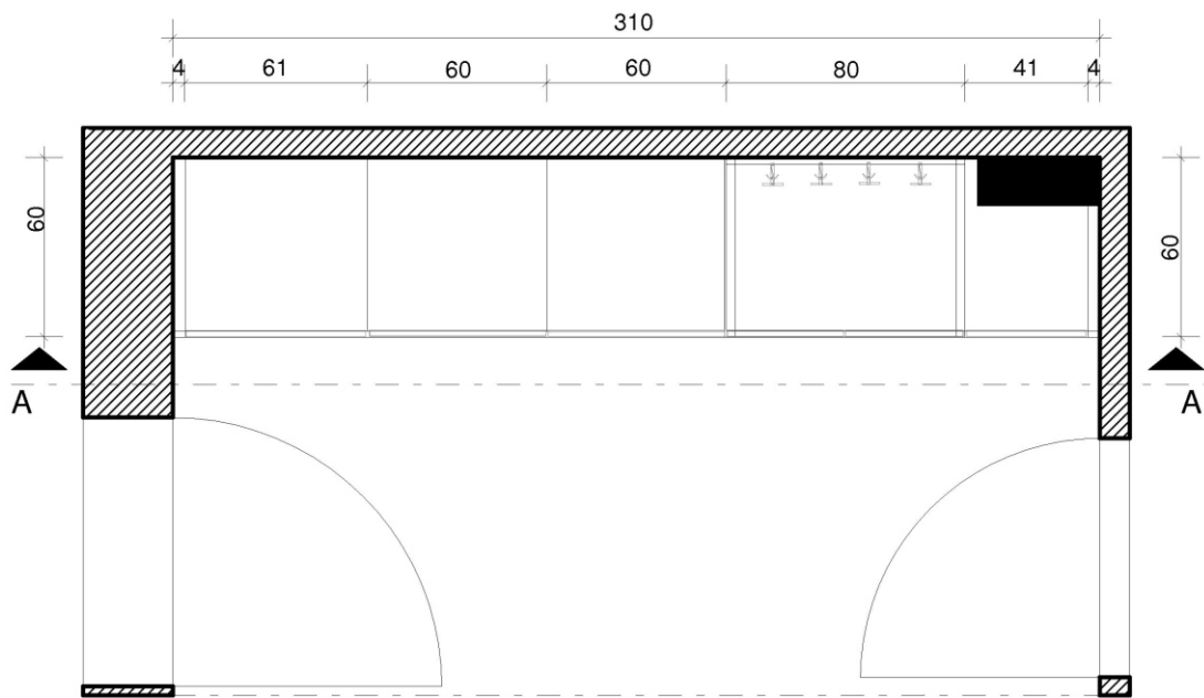
Řez A--A
