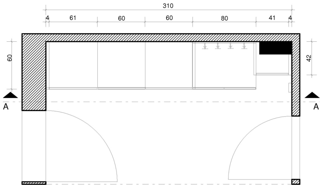
Řez A--A
