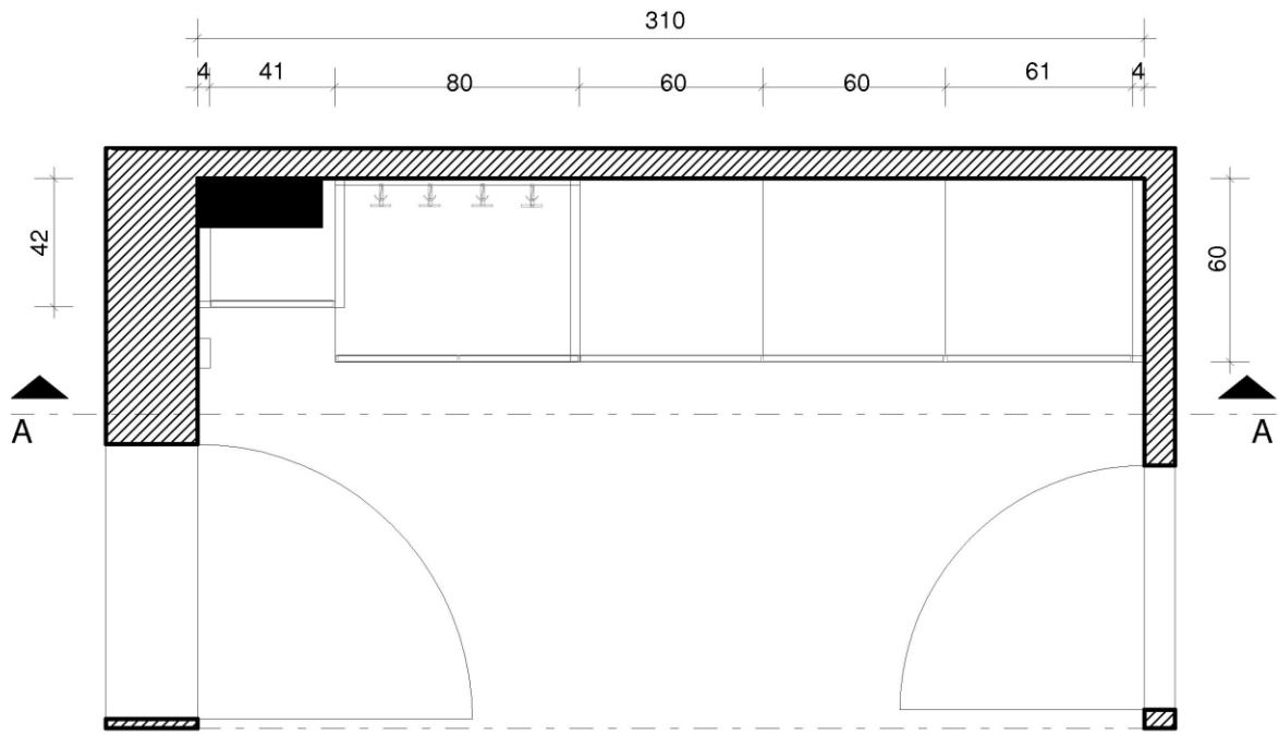
Řez A--A
