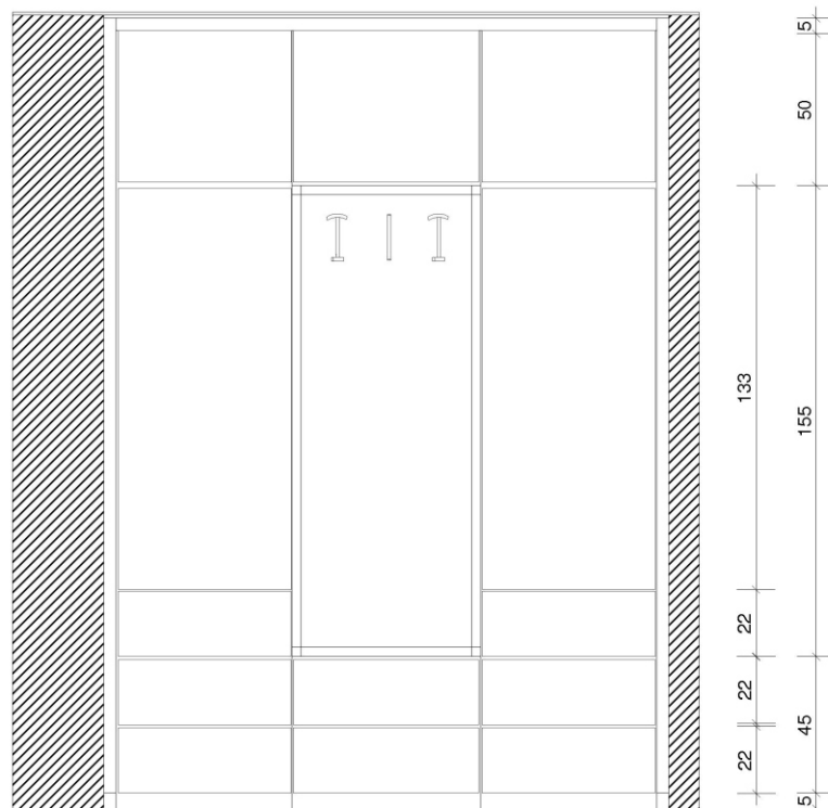
Řez A--A
