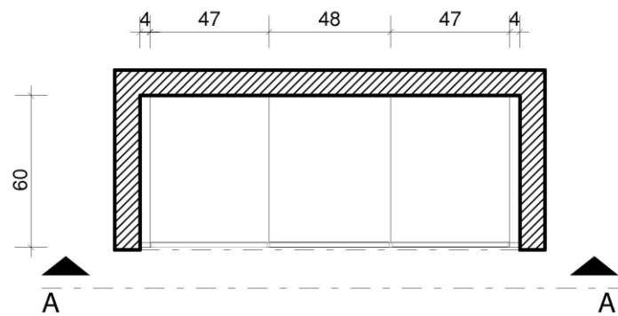
Řez A--A
