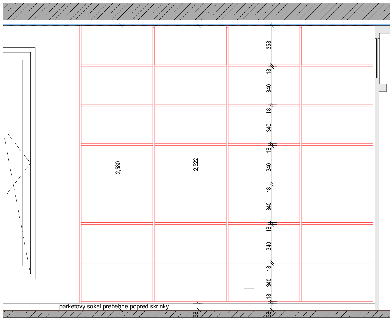
Pohľad satník 01 1:20
