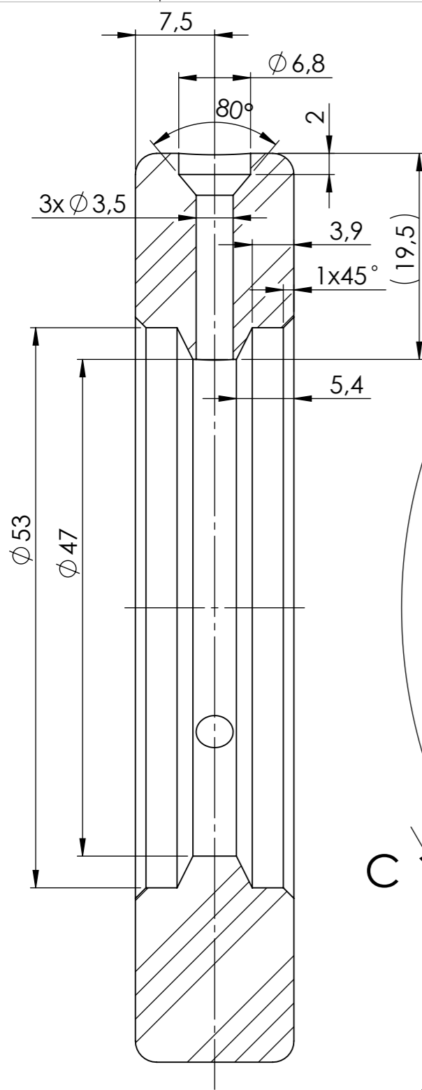
ŘEZ B-B MĚŘÍTKO 2:1
