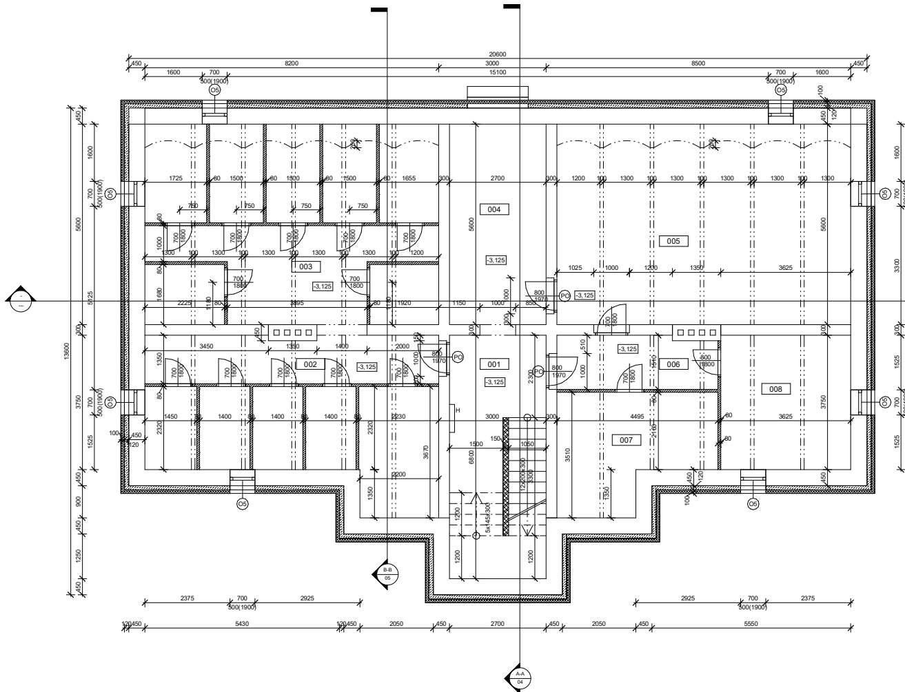
Výkaz místností_JifetIn - 1.PP
