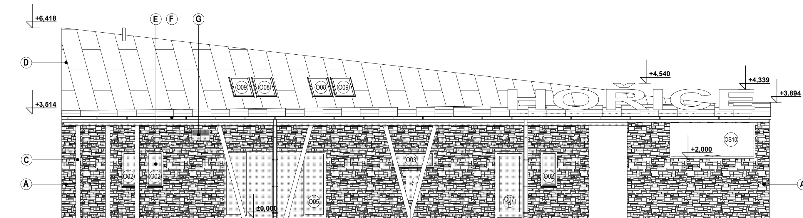
POHLED JIŽNÍ
