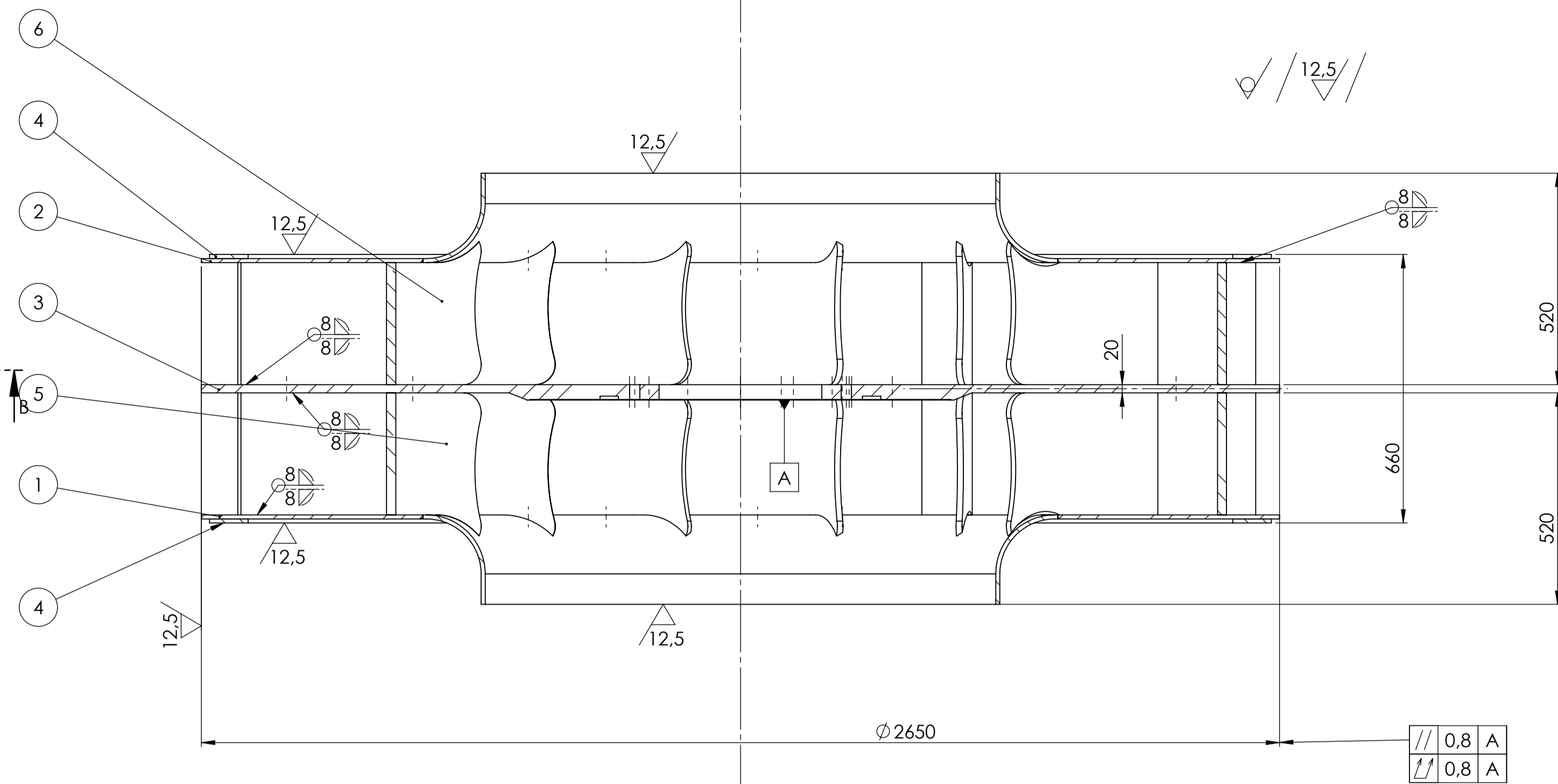
ŘEZ A-A MĚRITKO 1 : 10
