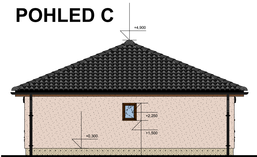
POHLED D
