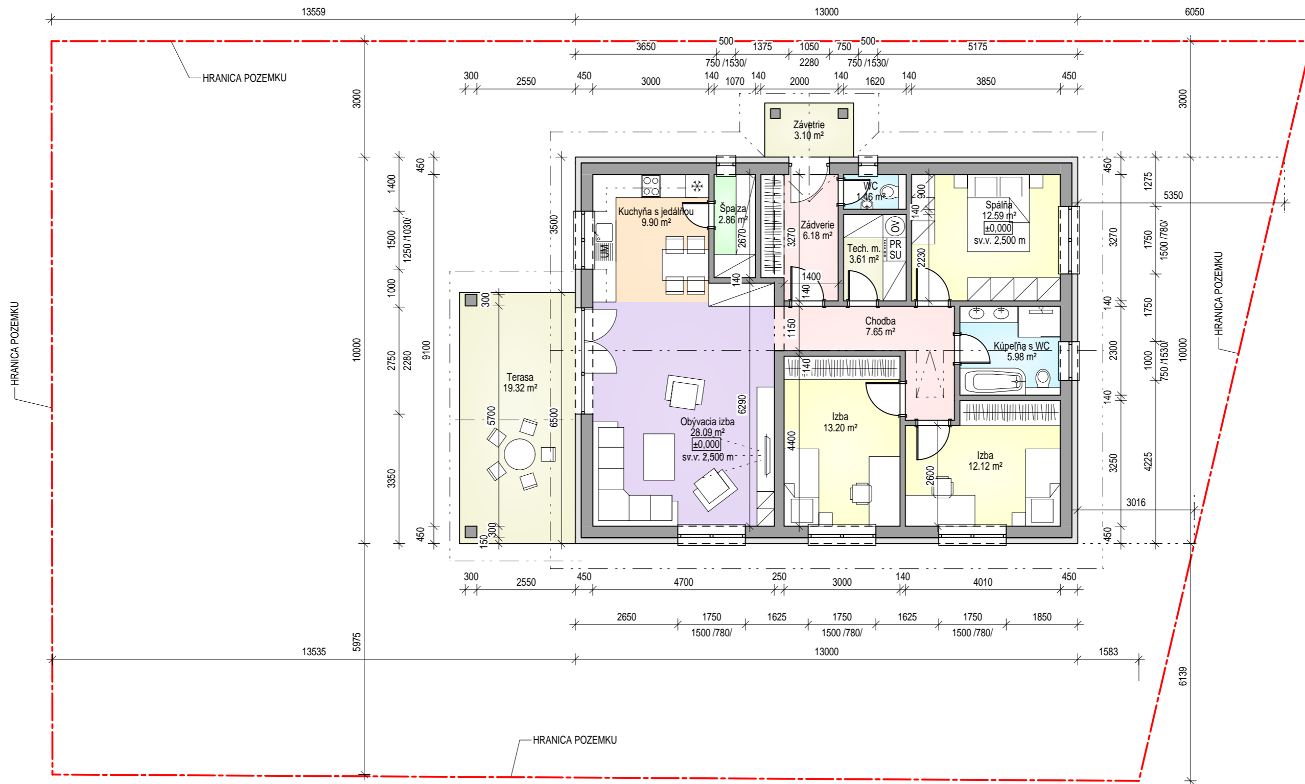
PÔDORYS 1.N.P. M1:100
