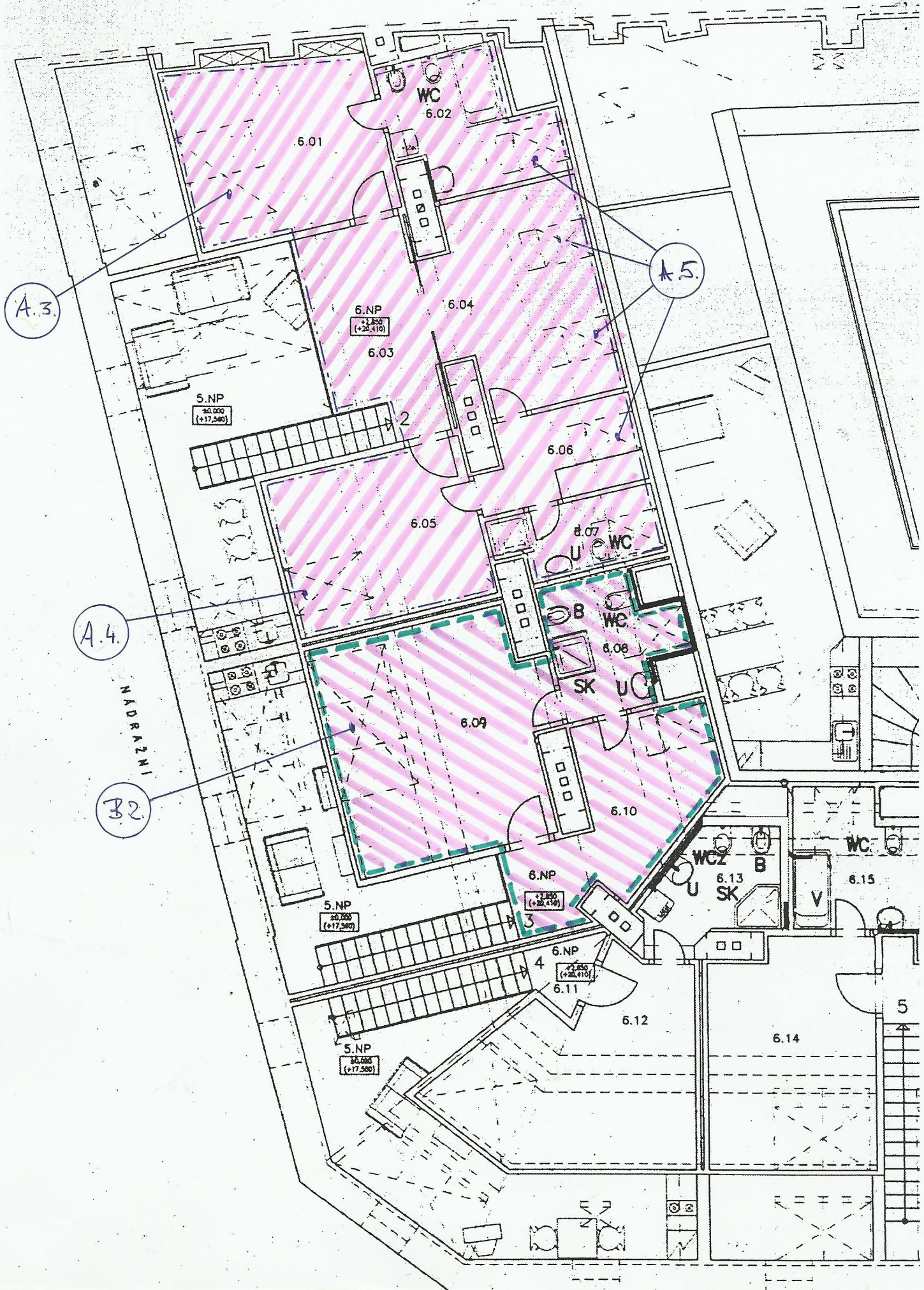
Příloha 2. - dispozice mezonetových bytů 6.N.P.
