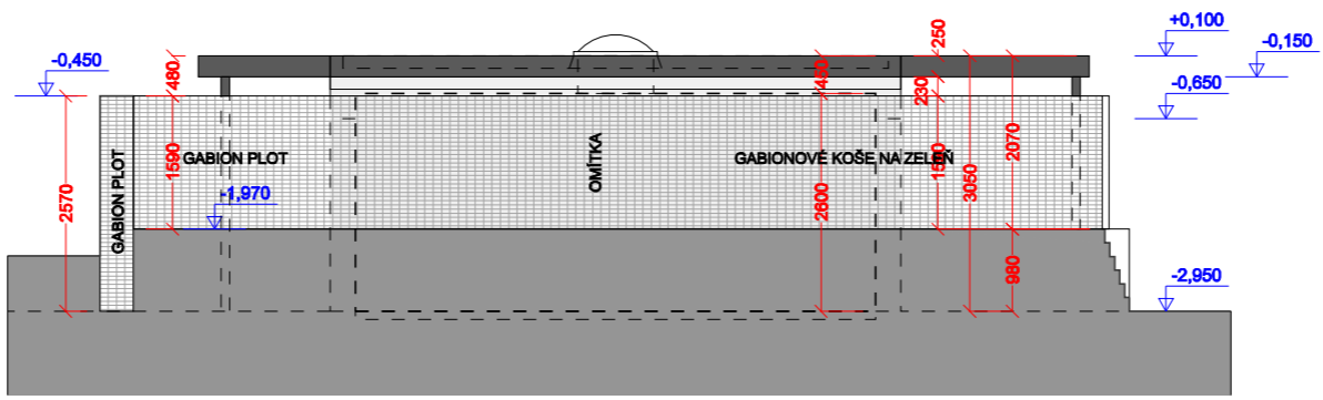
NÁVRH JIHOZÁPADNÍ POHLED - OD SOUSEDA
