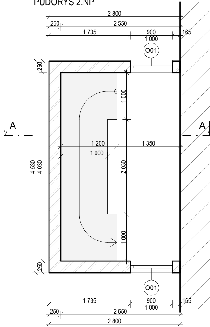
PŮDORYS 2.NP
