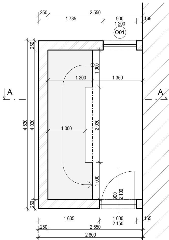
PŮDORYS 1.NP
